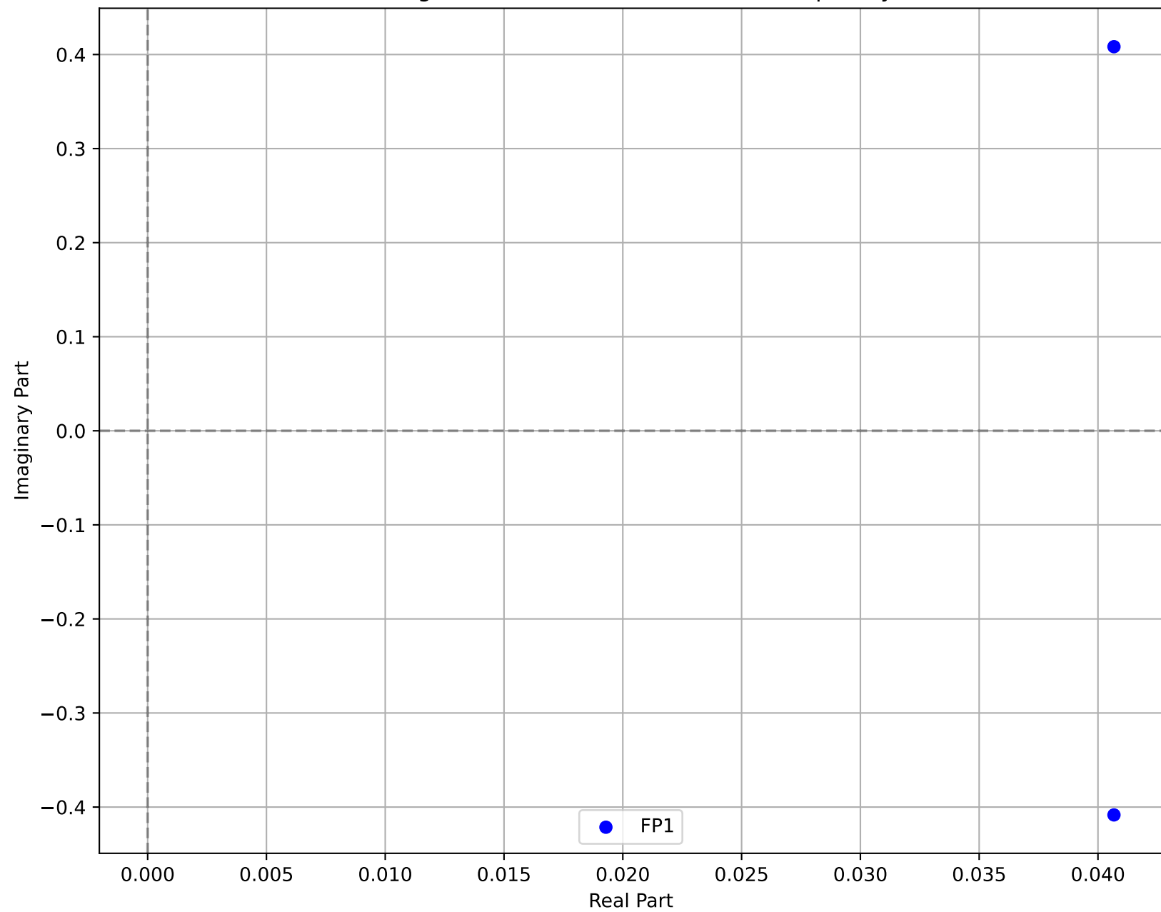
Unstable Eigenvalues for Task 25 ( \omega=0.350 , Sparsity=0.00)
