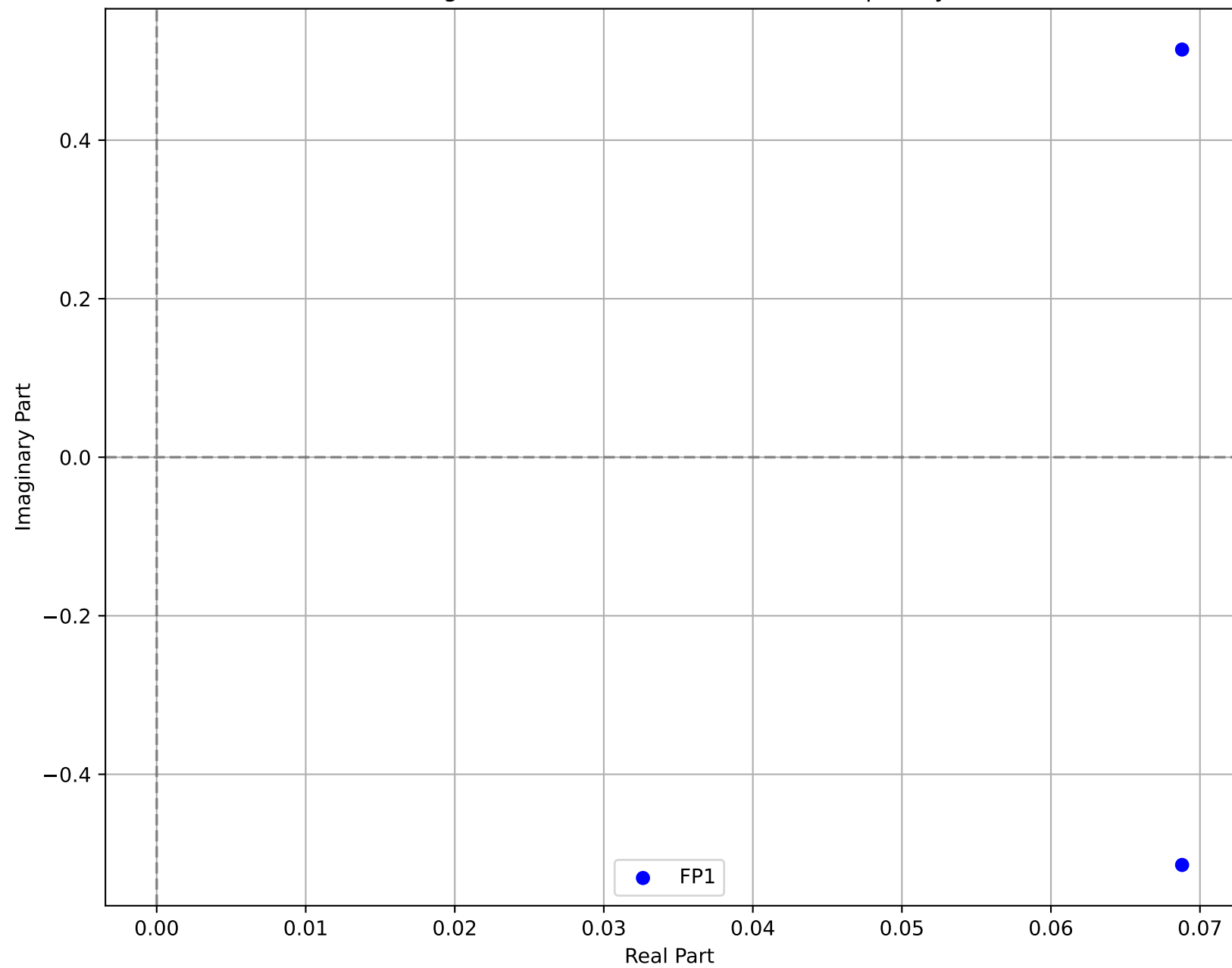
Unstable Eigenvalues for Task 37 ( \omega=0.470 , Sparsity=0.00)
