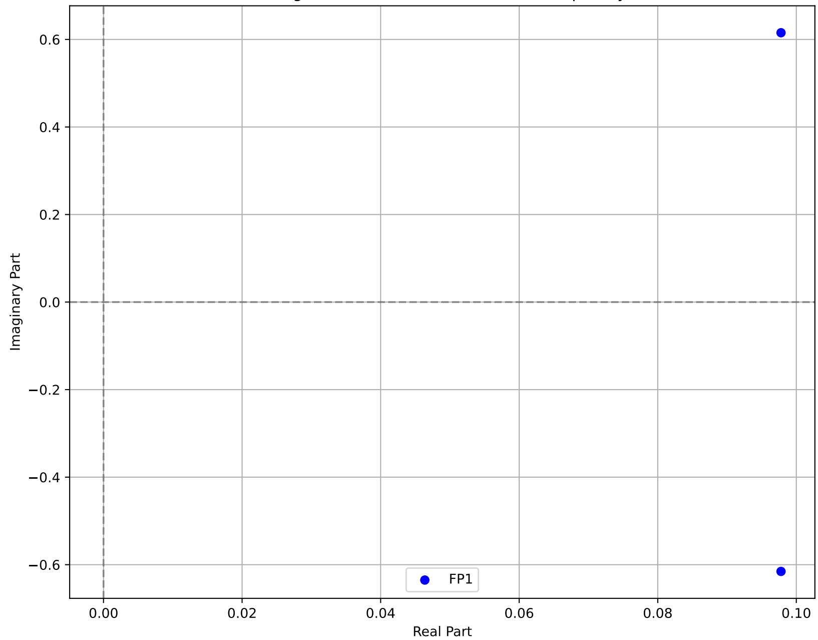
Unstable Eigenvalues for Task 50 ( \omega=0.600 , Sparsity=0.00)
