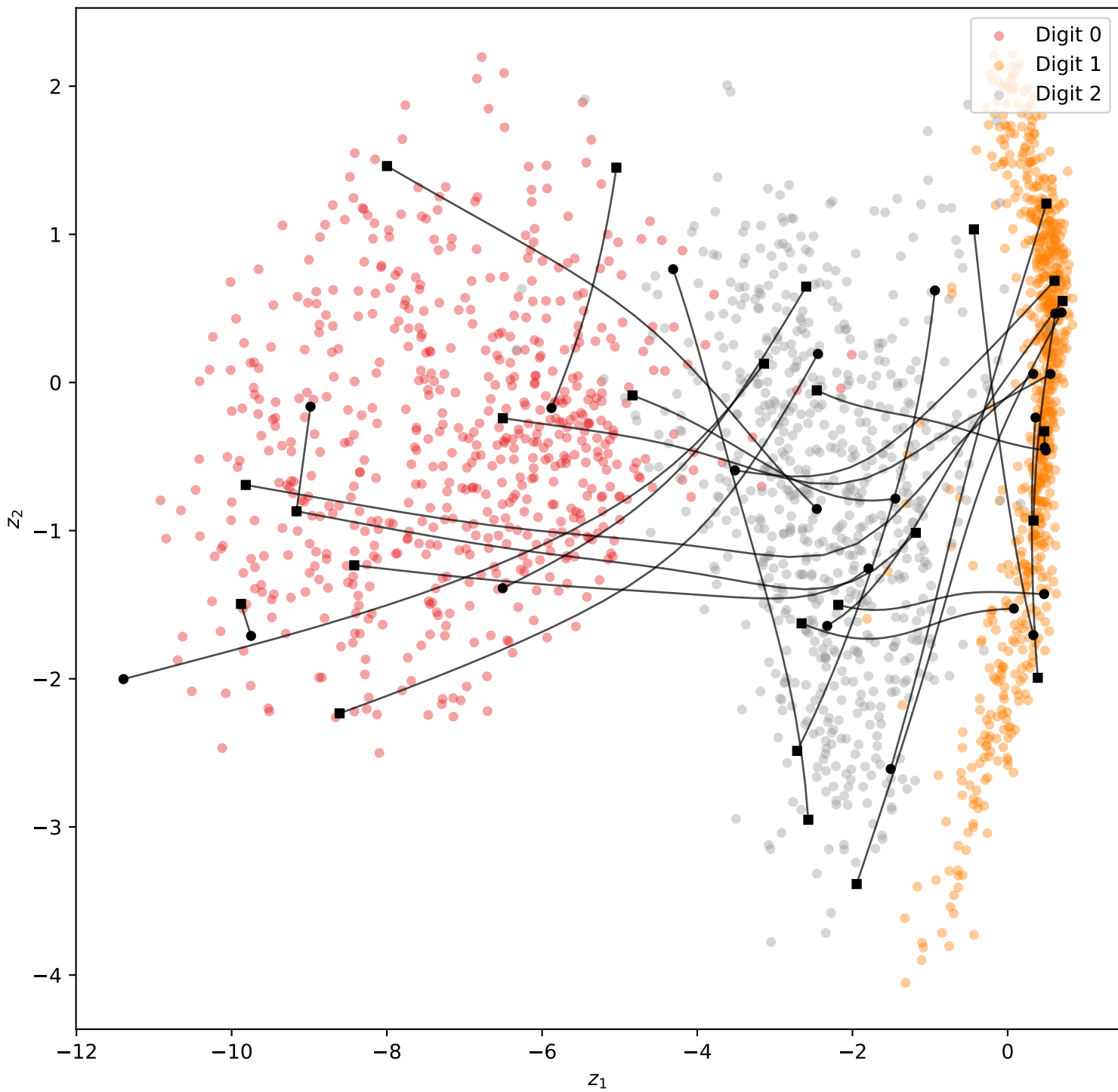
Geodesics (K=1 decoder)
