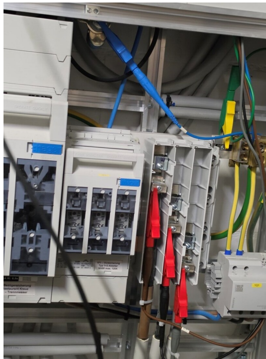
Bild 03 — Vorsicherung 1F1 mit Spannungsabgriffen
