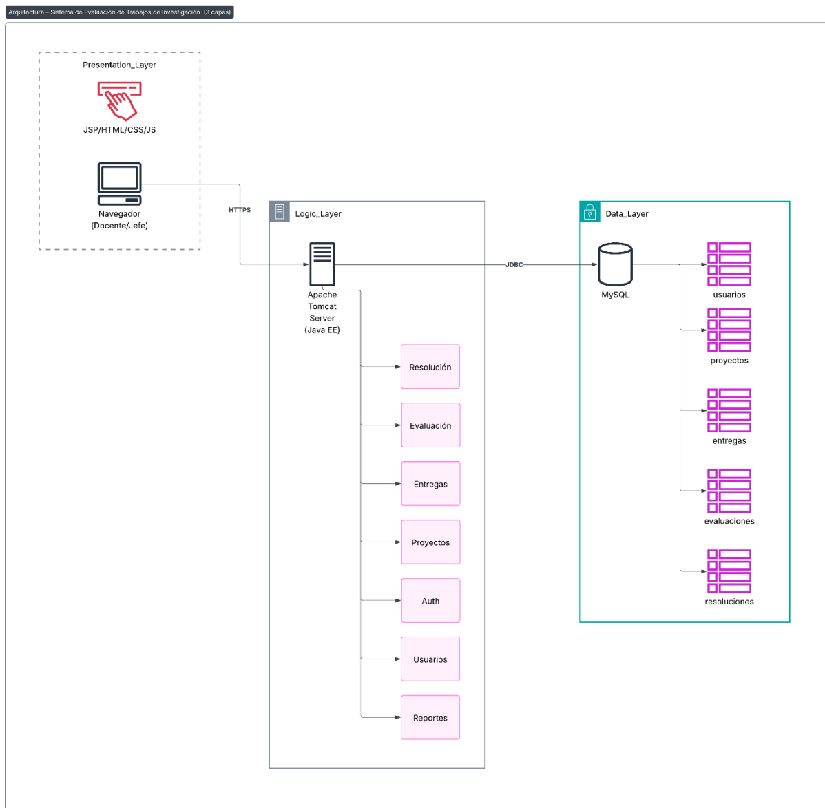
Figura 1. Diagrama de Arquitectura del Sistema.
