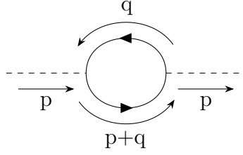
Figura 5.8: Self energia del campo scalare
