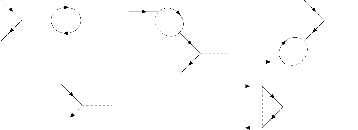
Figura 5.6: I contributi al secondo ordine perturbativo al vertice \bar{\psi}\psi\phi
