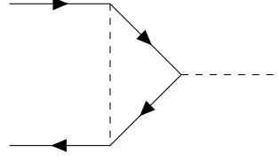
Figura 5.9: Diagramma a triangolo che contribuisce a \Gamma_{\bar{\psi}\psi\phi} al secondo ordine perturbativo
