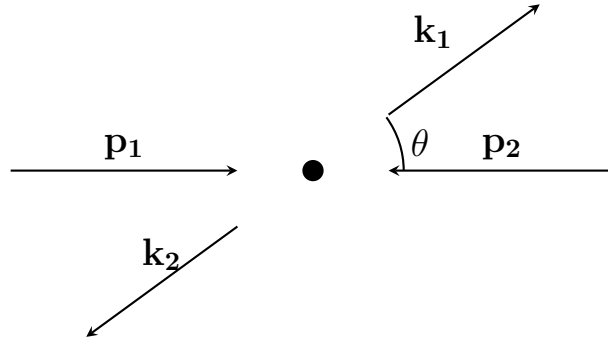
Figura 5.2: Scattering 2 \rightarrow 2 nel sistema del centro di massa.
