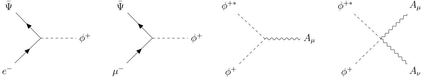
Figura 5.10: Nuovi vertici aggiunti dall'estensione
