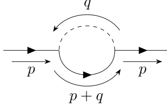
Figura 5.7: Contributo ad 1 loop della funzione a due punti del campo spinoriale
