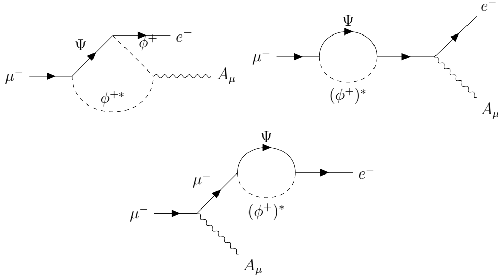
Figura 5.11: Diagrammi di Feynman per il decadimento \mu^- \rightarrow e^- \gamma
