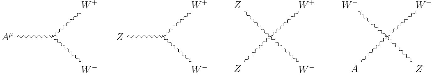
Figura 4.3: Esempi di possibili diagrammi di Feynman fra bosoni di gauge
