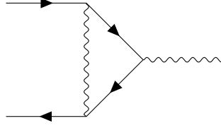
Figura 3.2: Il vertice ee\gamma considerando tutti i contributi
