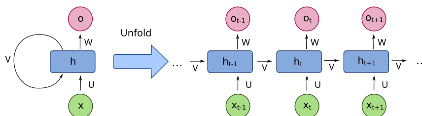
Figura 1.1: Rete Neurale Ricorrente e unfolding . Fonte: https://commons.wikimedia.org/w/index.php?curid=60109157
