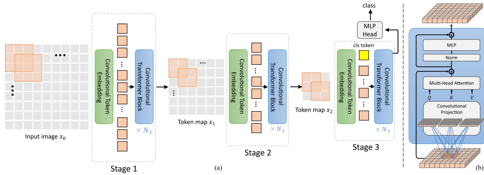
Figura 2.3: A sinistra l'architettura CvT, a destra la struttura del blocco Convolutional Transformer . Fonte: [28].
