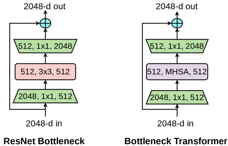
Figura 2.2: Confronto tra il blocco ResNet e il blocco BoTNet. Fonte: [21].
