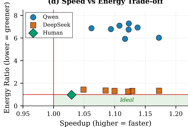
(d) Speed vs Energy Trade-off
