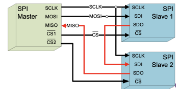
Abbildung 2: SPI-Topologien, Signale und Master-Slave-Prinzip.
