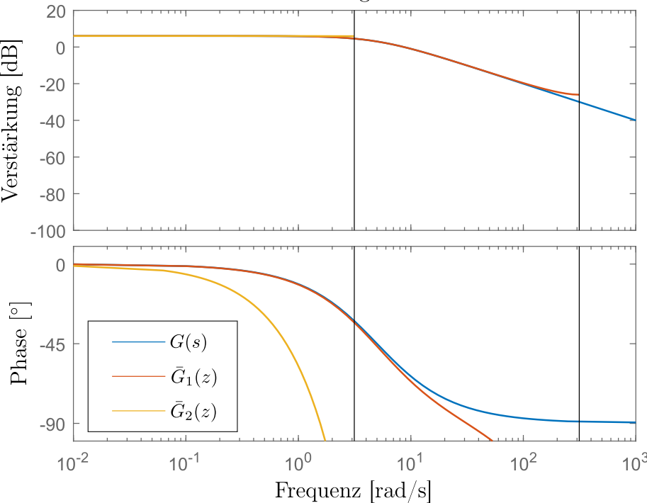
Bodediagramm
