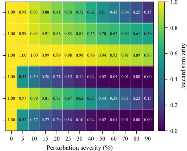
(b) FCC
