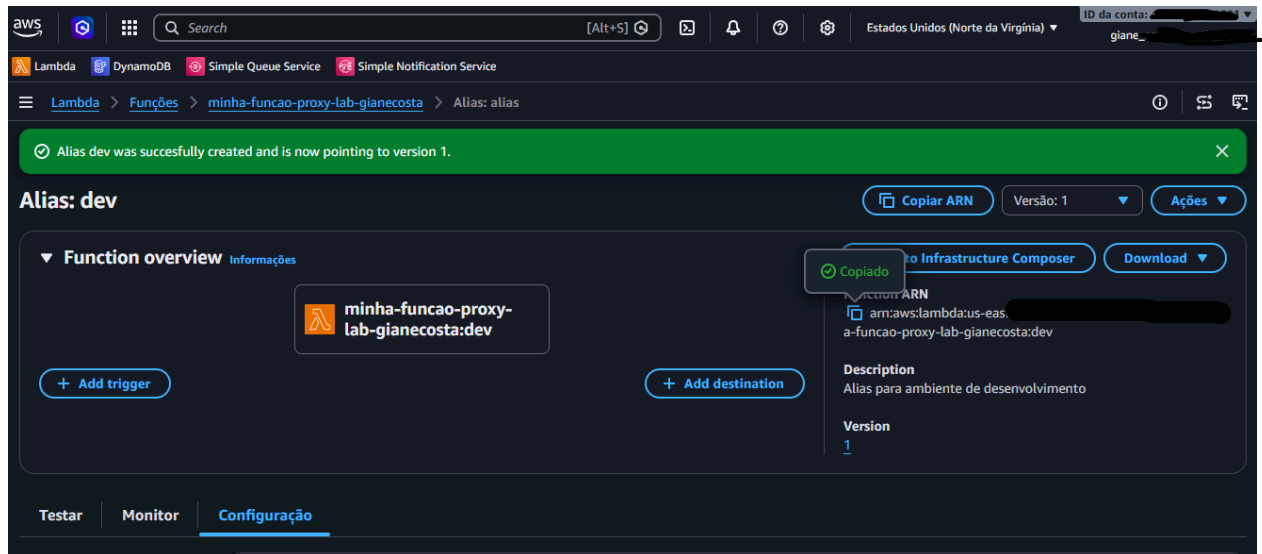
Imagem 1: Versão 1 e Alias dev configurado no AWS Lambda
