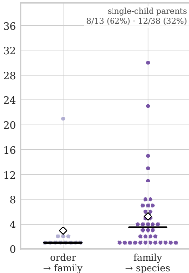
CUB-200
