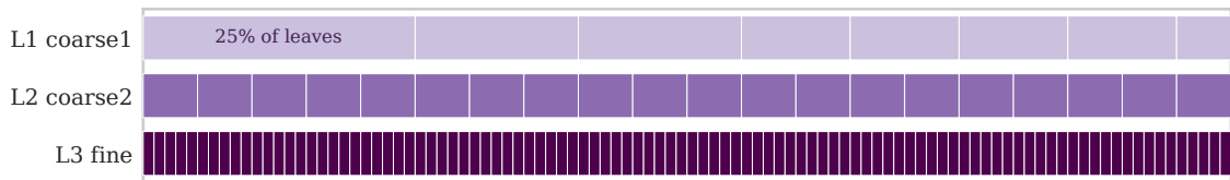
CUB-200 (13→38→200)
