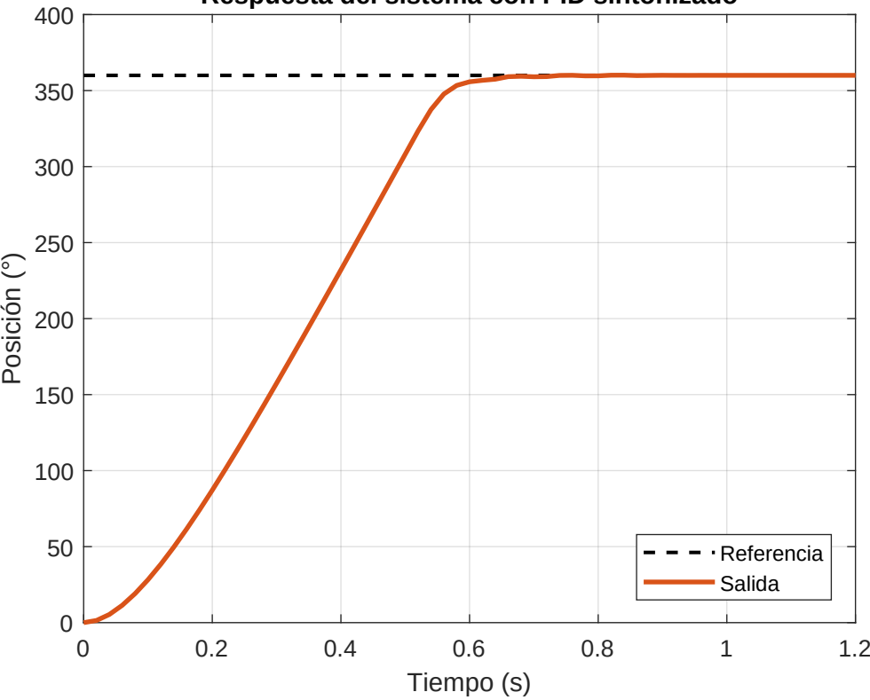
Respuesta del sistema con PID sintonizado
