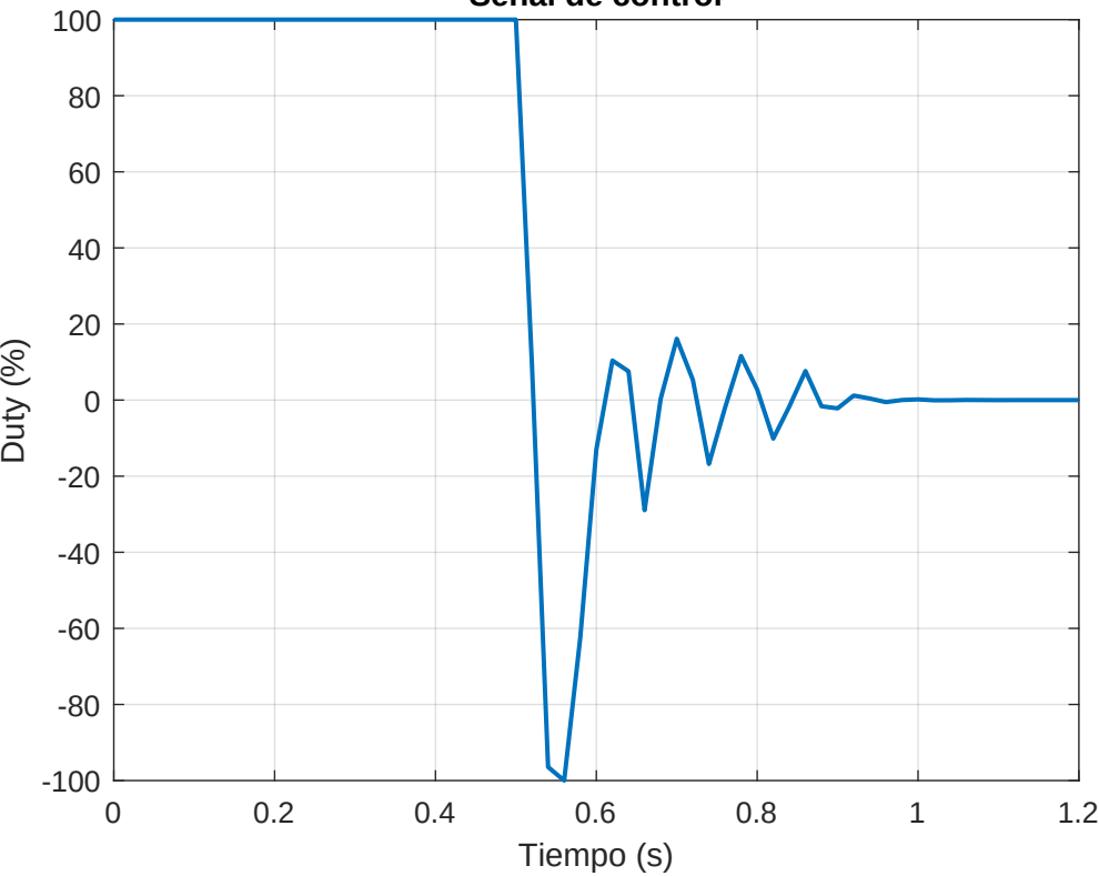
Señal de control
