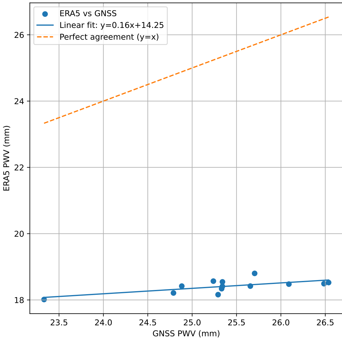
GNSS PWV vs ERA5 PWV - 22122025
