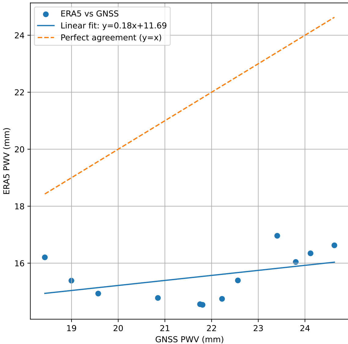
GNSS PWV vs ERA5 PWV - 24122025
