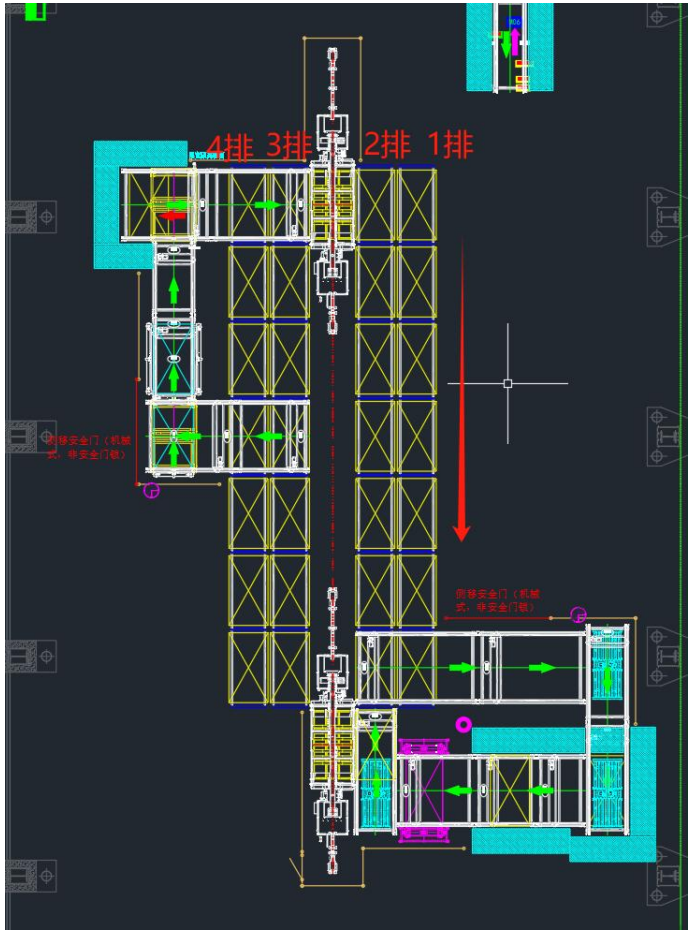
车架立体库，4排7列5层，其中6个货位被占用
