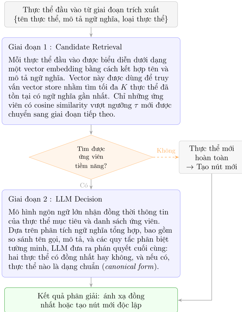
Hình 3.9: Kiến trúc hai giai đoạn của module phân giải thực thể. Giai đoạn Candidate Retrieval sử dụng embedding similarity để truy hồi các thực thể ngữ nghĩa tương đồng từ vector store. Giai đoạn LLM Decision chỉ được kích hoạt khi có ứng viên vượt ngưỡng \tau , giúp tiết kiệm chi phí gọi LLM cho những thực thể hoàn toàn mới.
