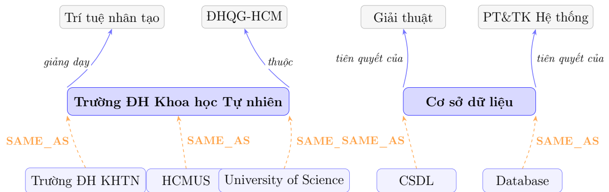
Hình 3.10: Ví dụ cấu trúc knowledge graph sau khi áp dụng phân giải thực thể trên corpus học thuật HCMUS. Các nút màu đậm là thực thể dạng chuẩn ( canonical ); các nút màu nhạt là hình thức tên thay thế ( alias ) được liên kết về nút chuẩn qua quan hệ SAME_AS (đường nét đứt cam). Quan hệ ngữ nghĩa thông thường (mũi tên xanh) chỉ xuất phát từ nút chuẩn, đảm bảo tri thức không bị phân tán.
