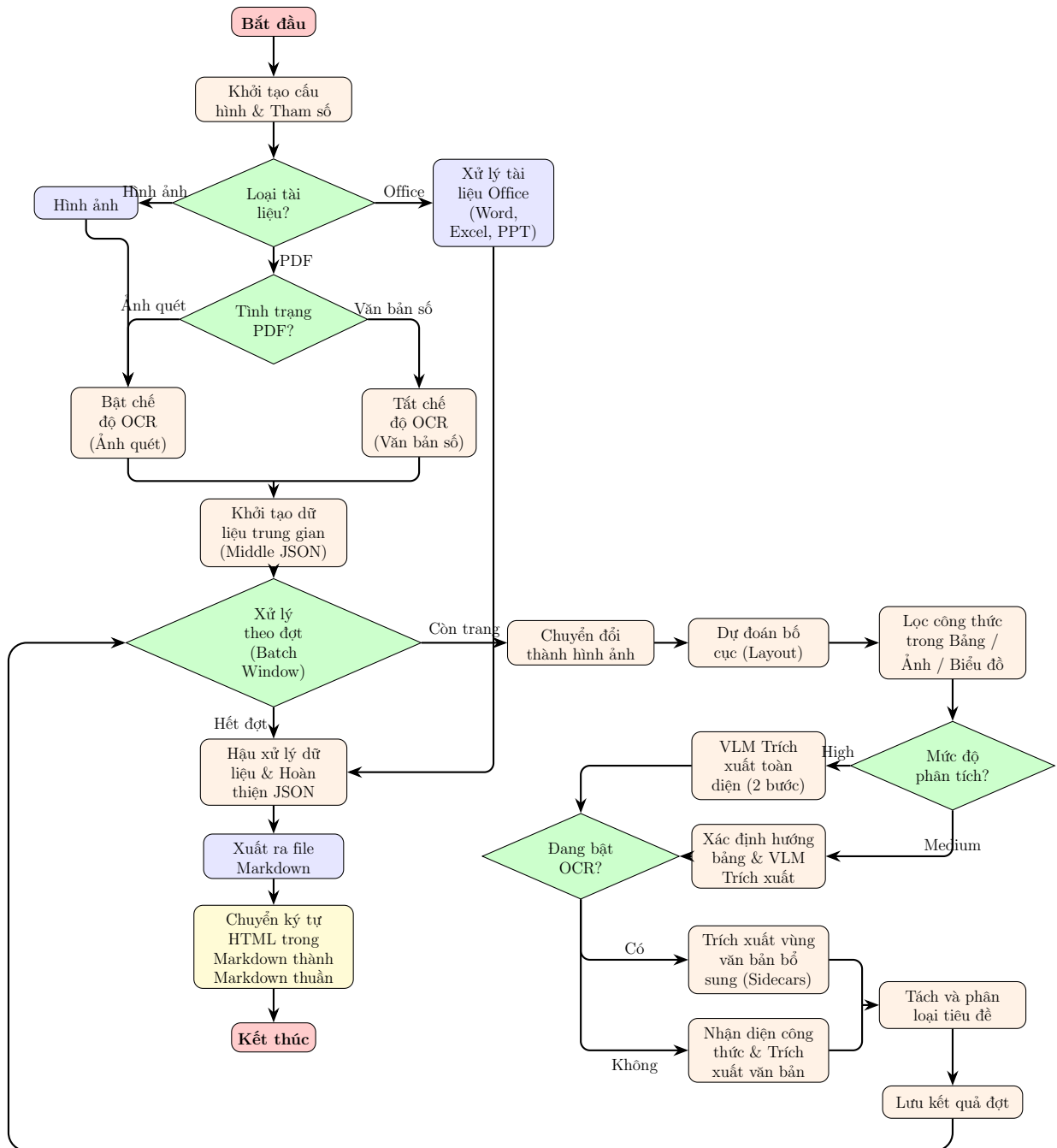
Hình 3.2: Quy trình Hybrid-Auto-Engine của MinerU[20]
