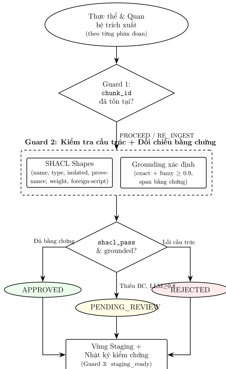
Hình 3.8: Quy trình kiểm chứng tri thức ba lớp bảo vệ (3-Guard) dựa trên SHACL và đối chiếu bằng chứng
