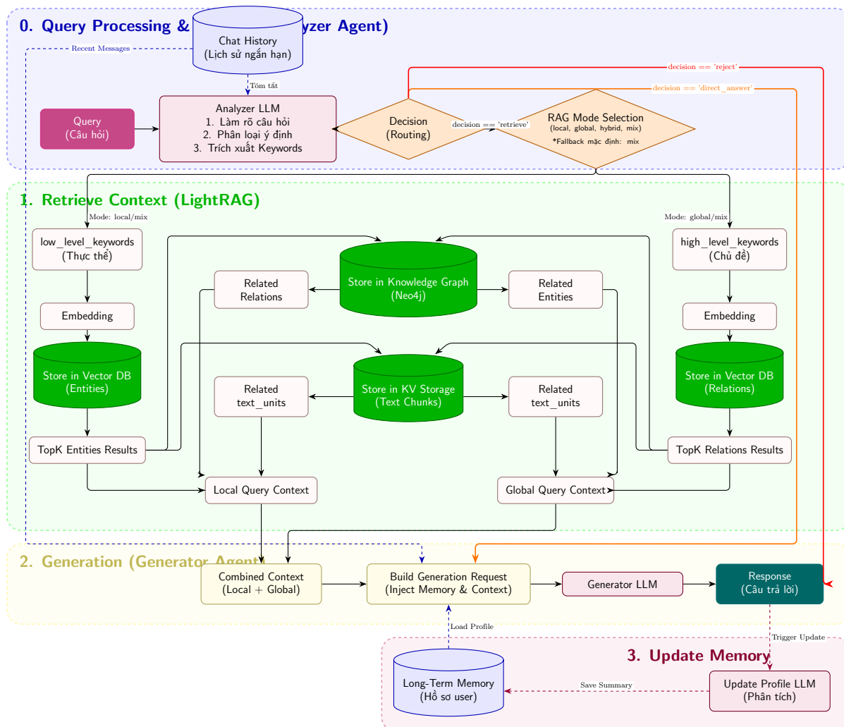
Hình 3.11: Quy trình truy vấn đa chế độ và cơ chế tối ưu phản hồi trong LightRAG
