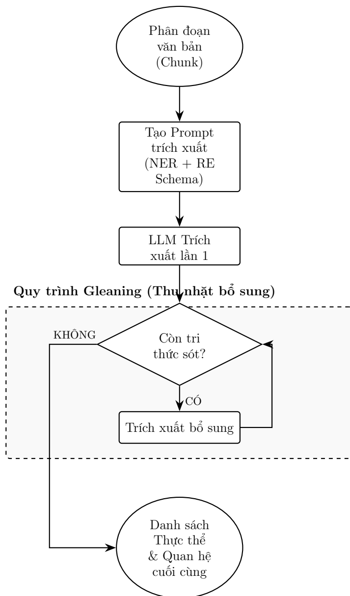
Hình 3.6: Luồng logic quy trình trích xuất tri thức và cơ chế Gleaning
