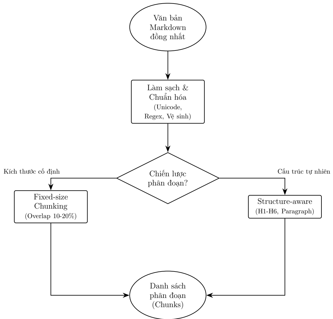
Hình 3.5: Luồng logic xử lý từ dữ liệu thô đến giai đoạn phân đoạn
