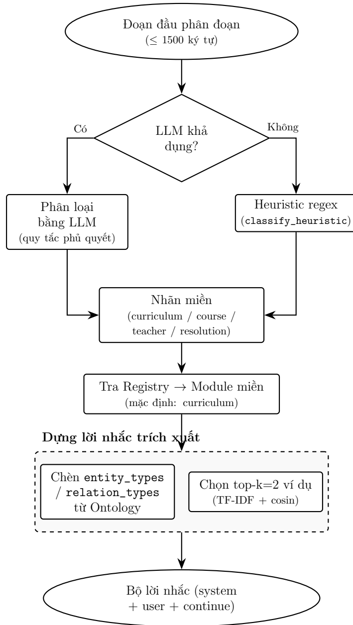
Hình 3.7: Luồng điều phối lời nhắc linh hoạt theo miền tri thức (Dynamic Prompt Flow)
