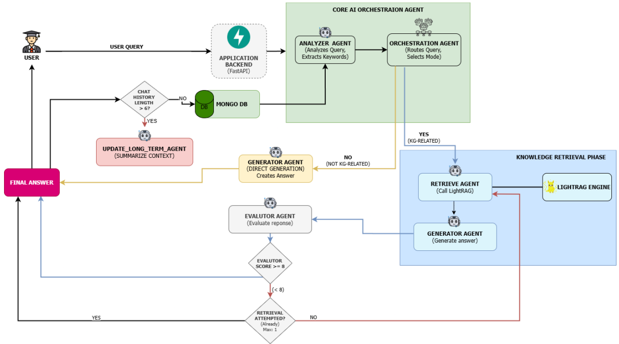
Hình 3.6: Sơ đồ quy trình xử lý query trong hệ thống ai agent
