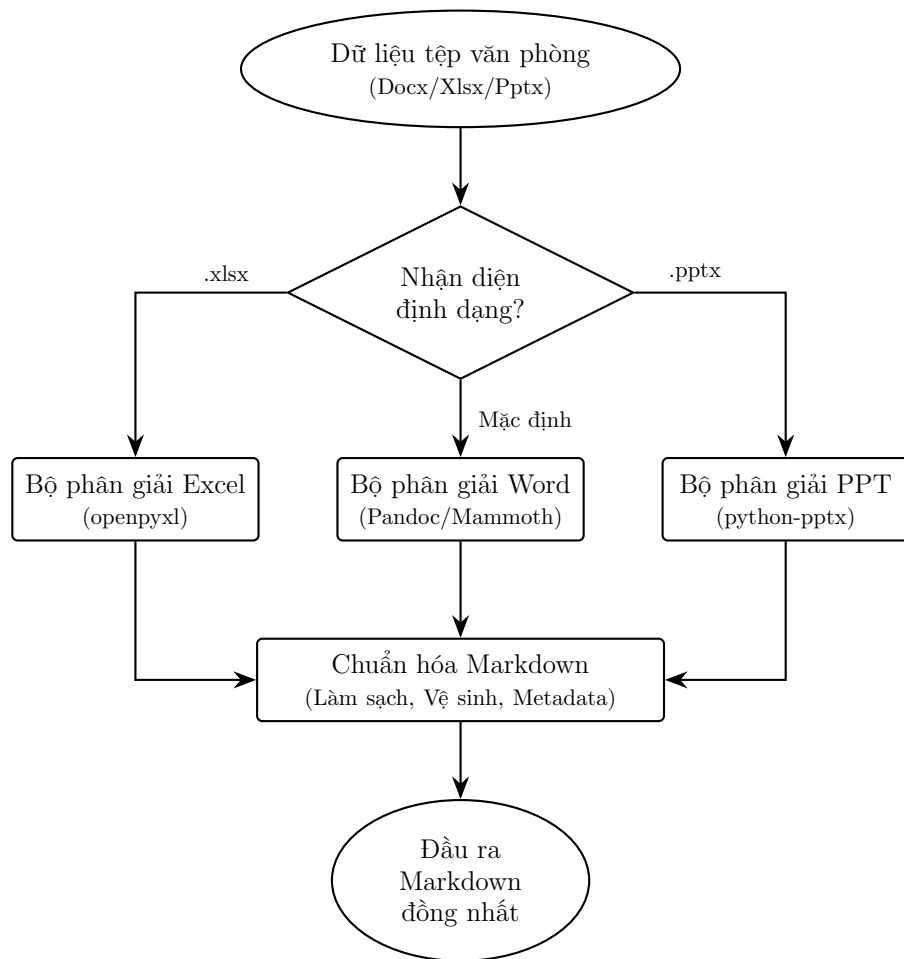
Hình 3.3: Sơ đồ hoạt động của hệ thống MarkItDown
