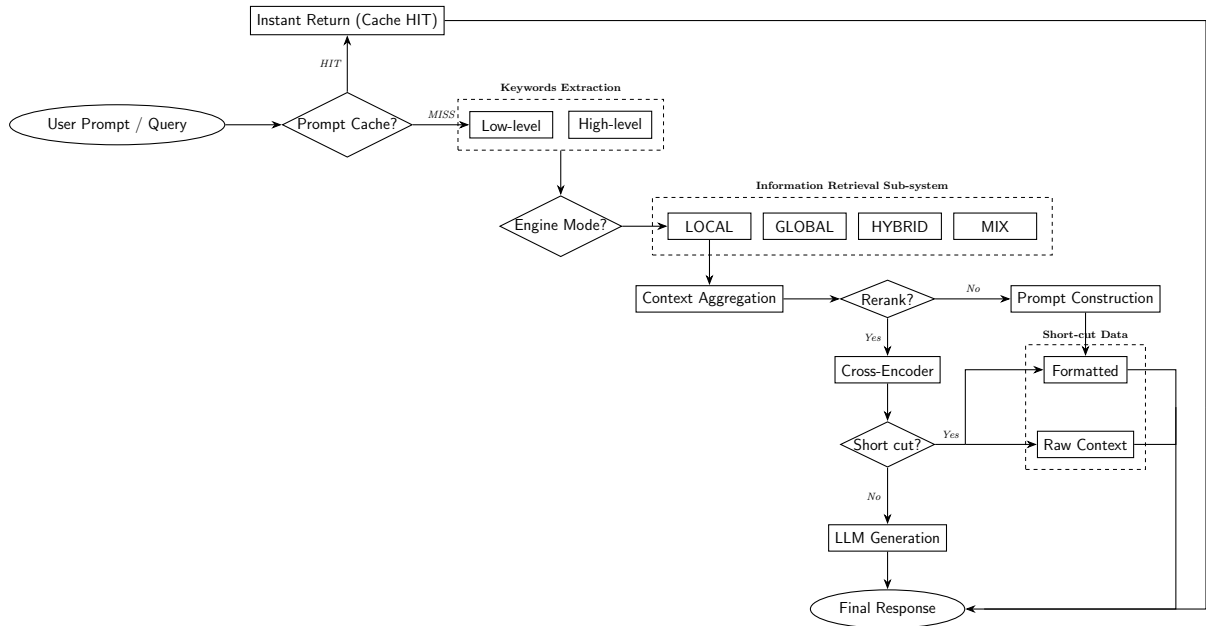
Hình 3.5: Quy trình truy vấn đa chế độ và cơ chế tối ưu phản hồi trong LightRAG
