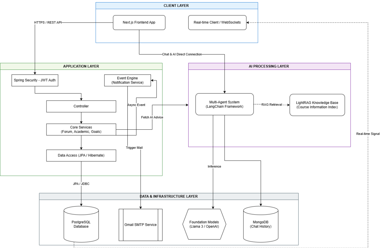
Hình 3.7: Mô hình kiến trúc hệ thống tổng thể
