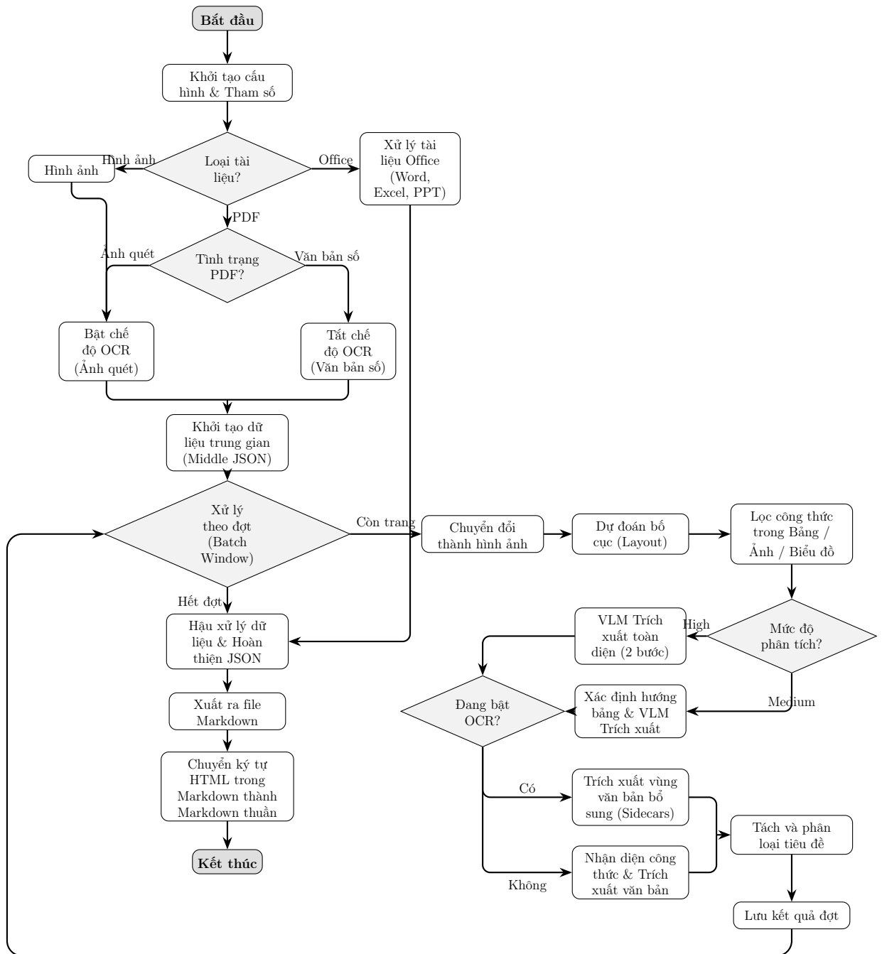
Hình 3.2: Quy trình Hybrid-Auto-Engine của MinerU[0]
