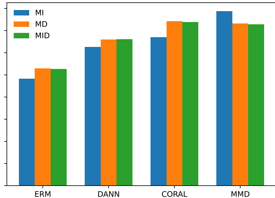
EEGConformer
