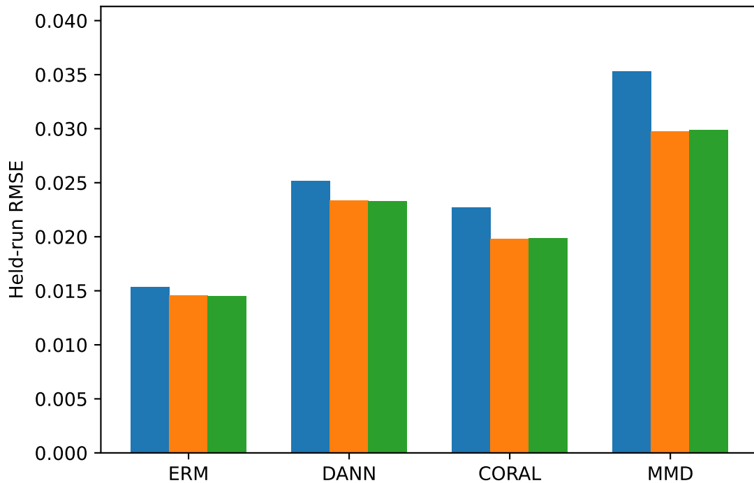
EEGNet
