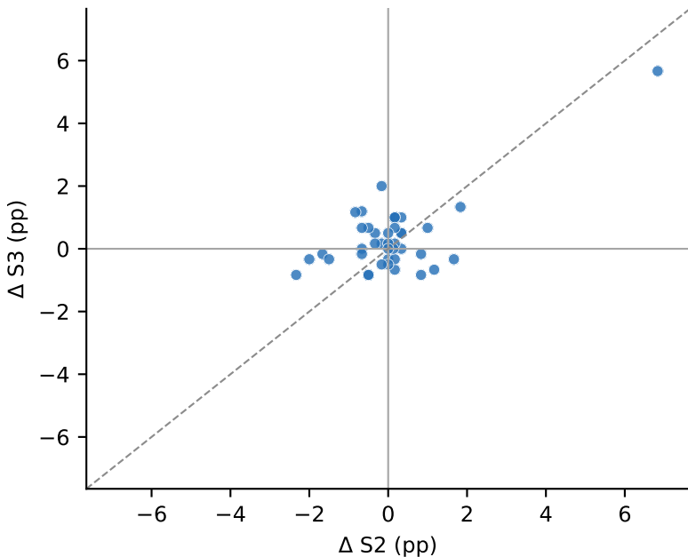
EEGNet (Spearman 0.18)
