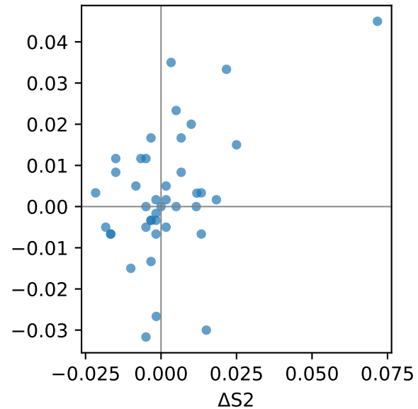
EEGConformer
