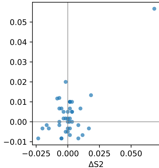
EEGNet
