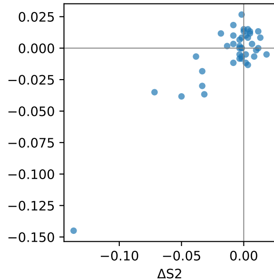
CBraMod
