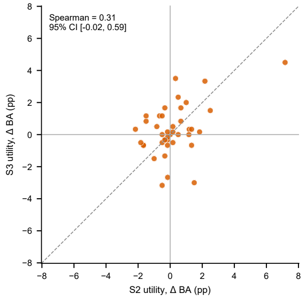
EEGConformer
