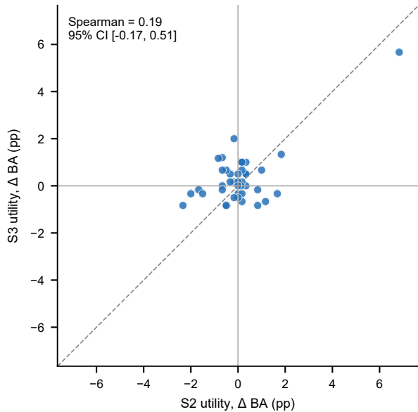
EEGNet
