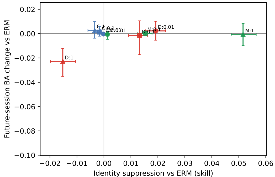
EEGNet
