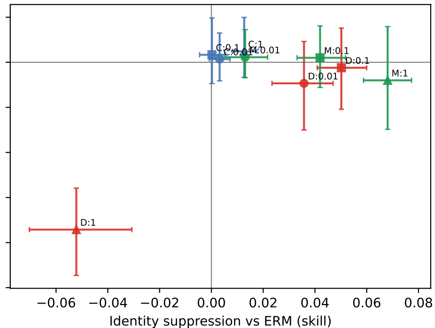
EEGConformer
