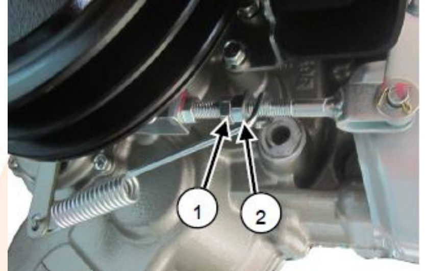
(1) Nati ya kufunga (2) Nati ya kurekebisha
