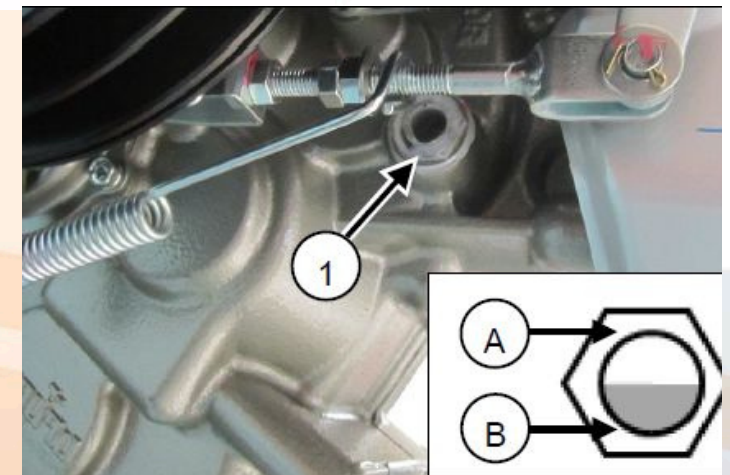
Kiwango cha mafuta ya upitishaji
