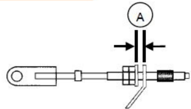
(A) Mchezo wa bure 3–5 mm
