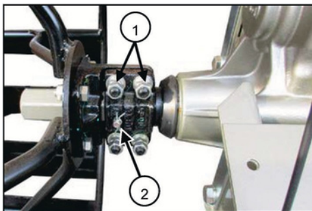
(1) Nati ya kufuli ya kitovu cha gurudumu (2) Pini ya kunasa na pini ya kitovu cha gurudumu
