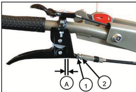
(1) Nati ya kufuli (2) Kirekebishaji (A) Kucheza bure kwa milimita 1-2
