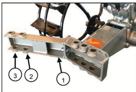
(1) Kifungo cha upanuzi (2) Shimo la jembe la diski (3) Shimo la jembe la ubao wa kuongoa
