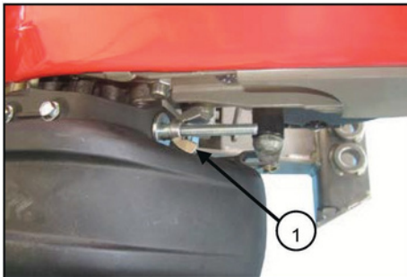
(1) Boliti ya kurekebisha mvutano wa mkanda
