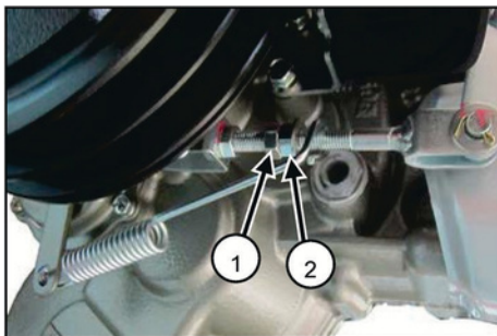
(1) Nati ya kufunga ya kurekebisha breki (2) Nati ya kurekebisha breki
