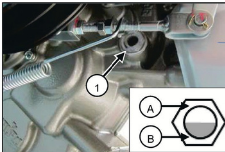
(1) Lango la kukagua kiwango (A) Kiwango cha juu zaidi (B) Kiwango cha chini zaidi
