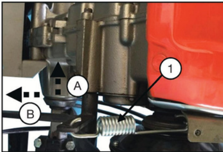
(1) Chemchemi (A) Upande wa koili ya chemchemi (B) Upande wa mbele wa kutembea nyuma trekta
