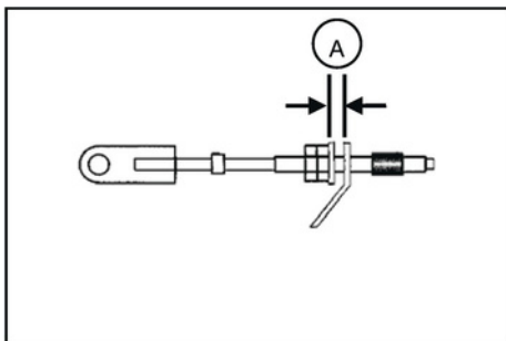
(A) Michezo wa bure wa breki kwenye
