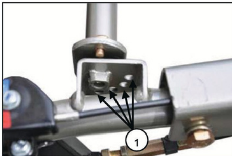
(1) Shimo la kurekebisha sehemu ya kushikilia kipini
