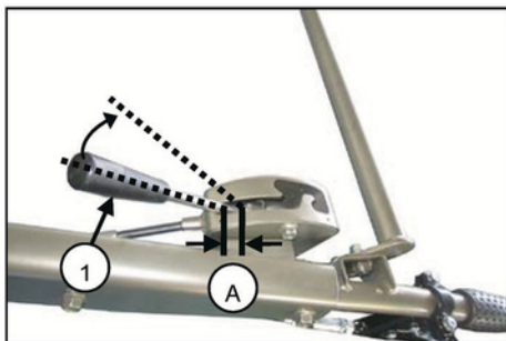
(1) Kifaa kikuu cha clutch (A) Mchezo huru
