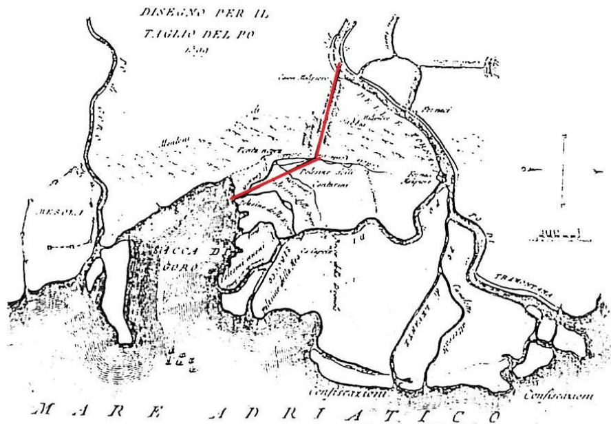
Bernardino Zendrini "Memorie Storiche delle Lagune Venete" Tavola XX - Tomo I Disegno del Taglio del PO (1600)
