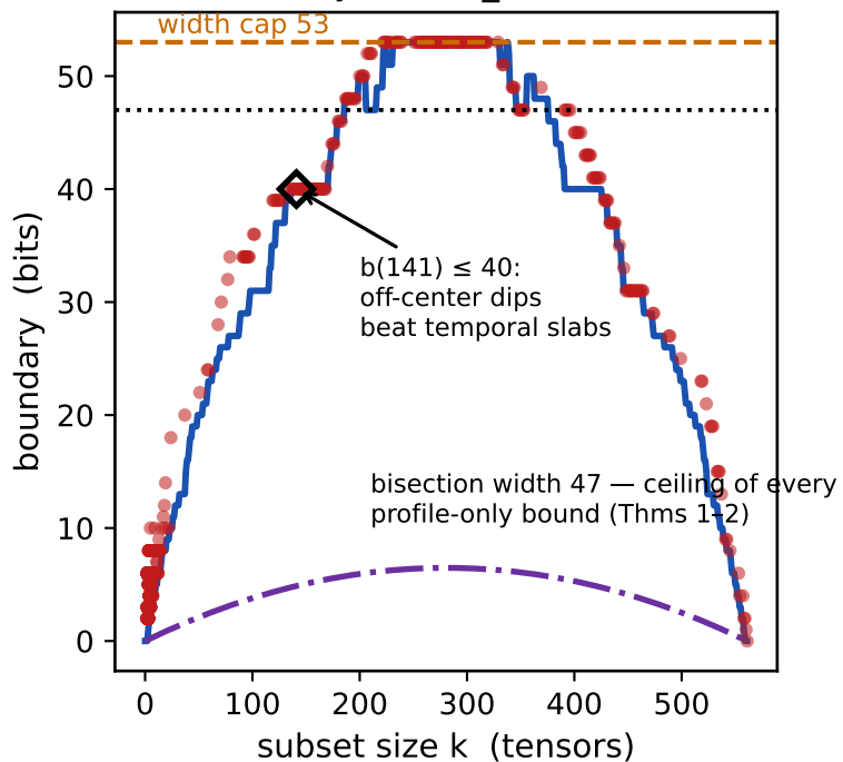
sycamore_m20
