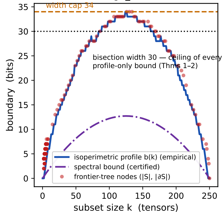
reg3_250
