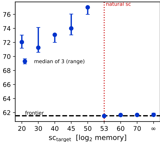
sycamore_m20
