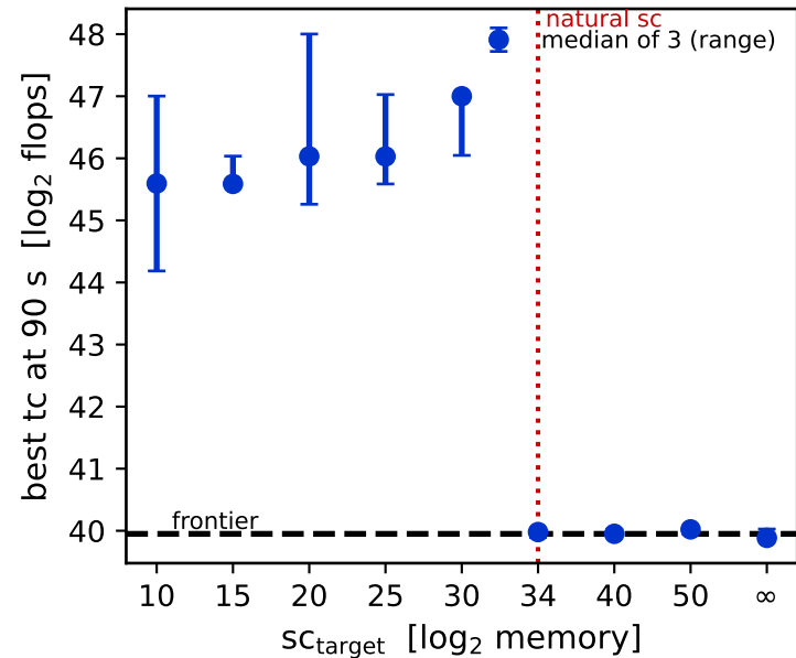
reg3_250
