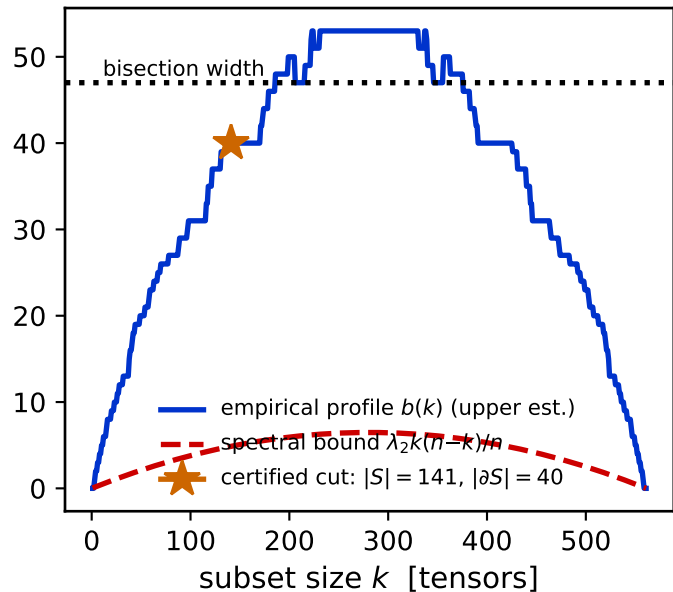
sycamore_m20
