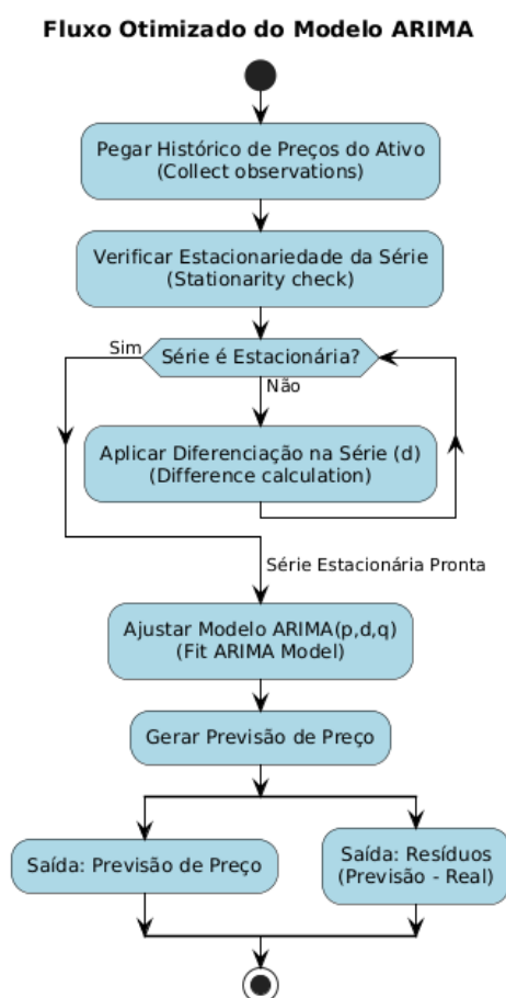
Figura 5 – Fluxo ARIMA
