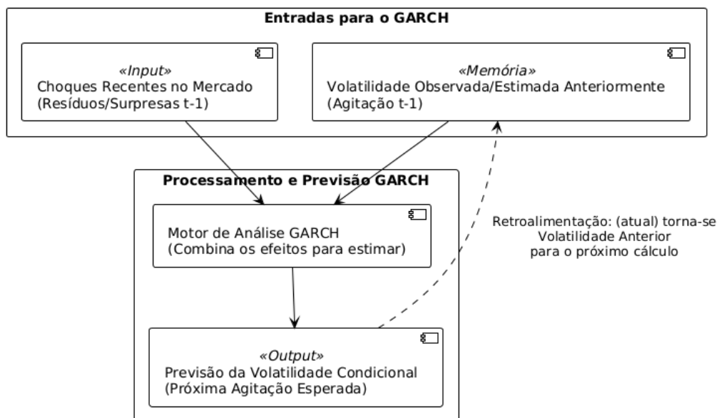
Figura 6 - Fluxo GARCH
