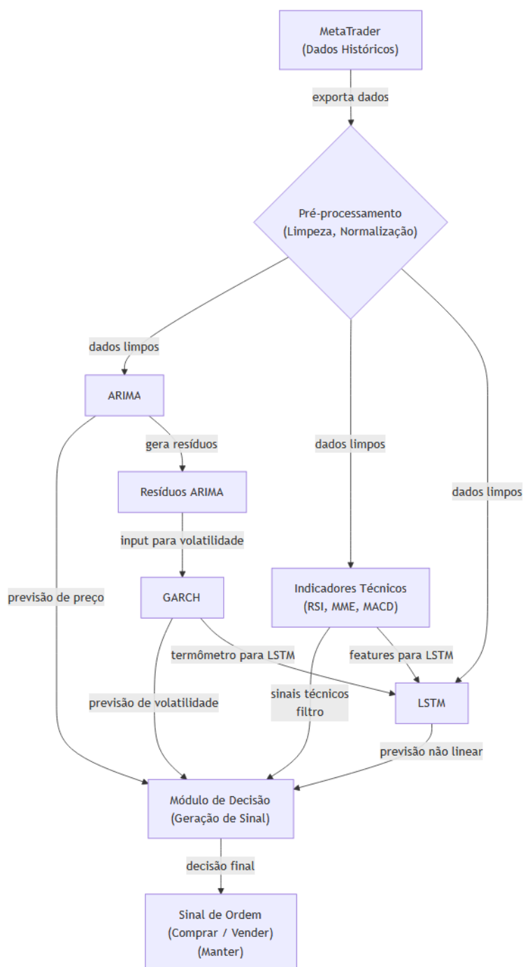
Figura 7 - Fluxograma Completo
