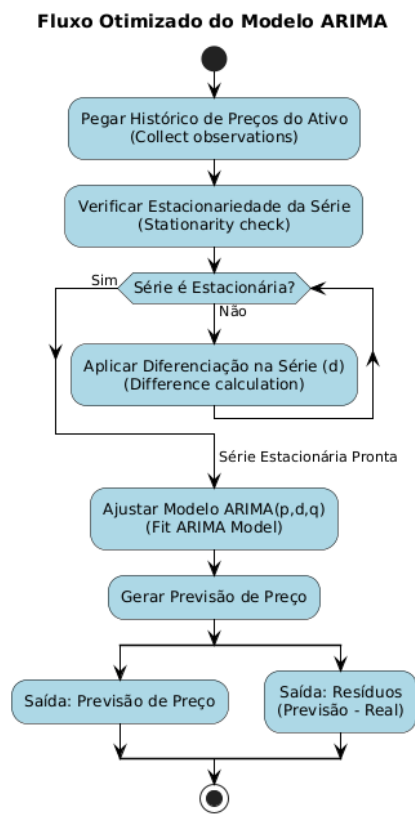
Figura 5 - Fluxo ARIMA
