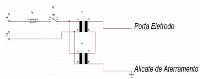
Figura 2: Esquema elétrico máquina de solda a ponto
