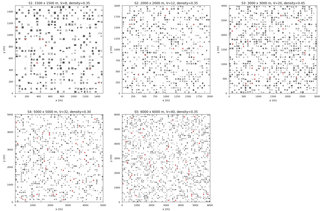
그림 2. S1-S5 확장 시나리오별 도시 맵 및 버티포트 배치
