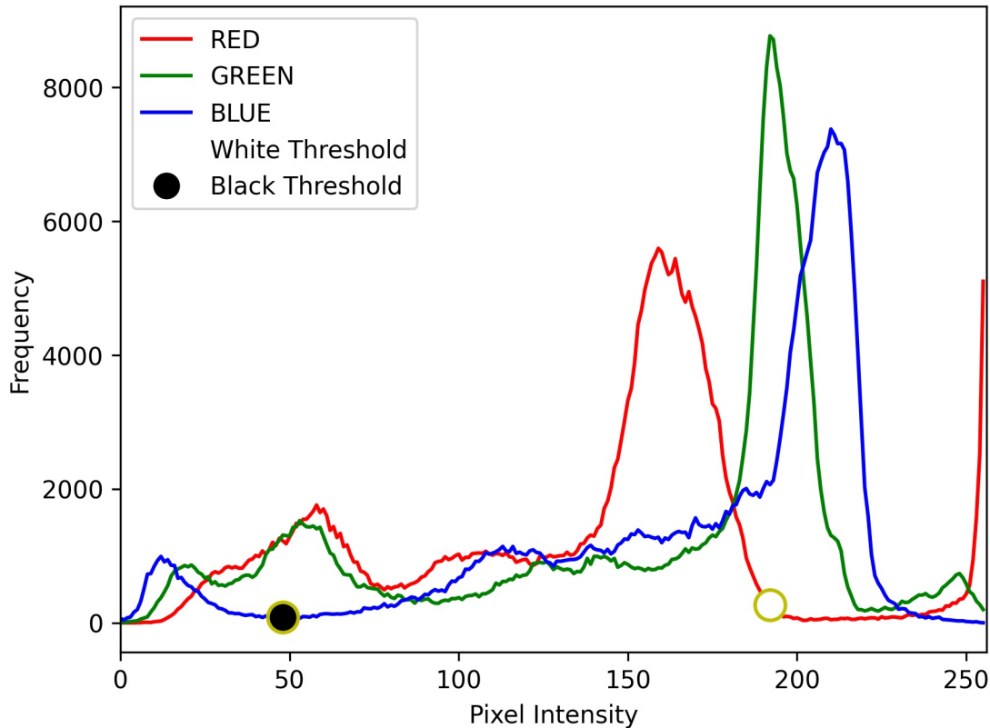
RGB Histogram
