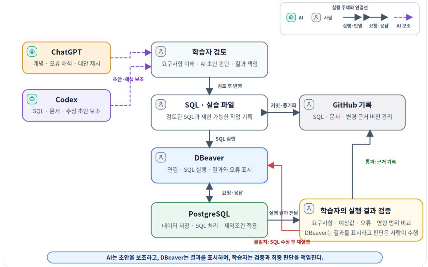
그림 3-1 전체 데이터베이스 작업 환경
