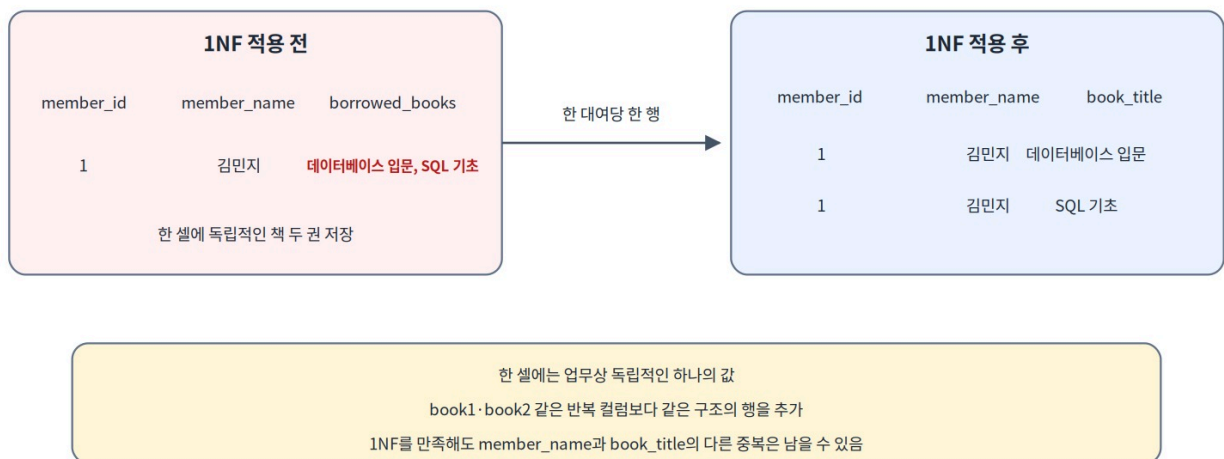
그림 6-3 제1정규형: 독립 값을 행으로 분리하기
