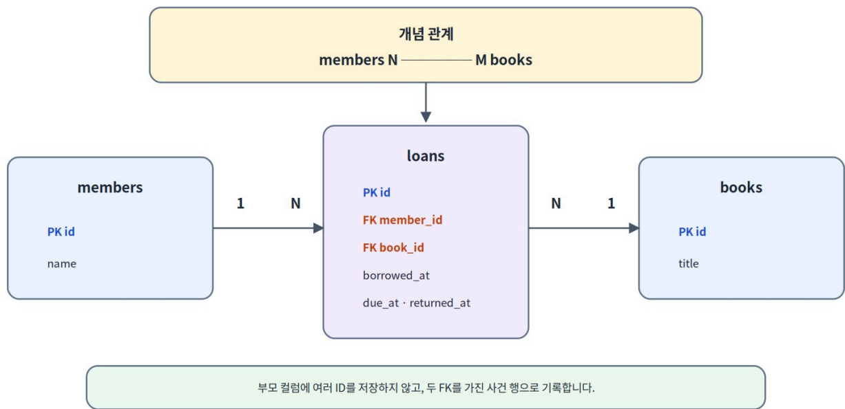
그림 5-3 N:M 관계를 사건 테이블로 풀기
