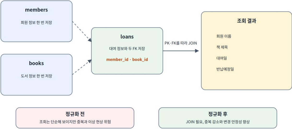
그림 6-7 정규화된 저장과 조회 결과
