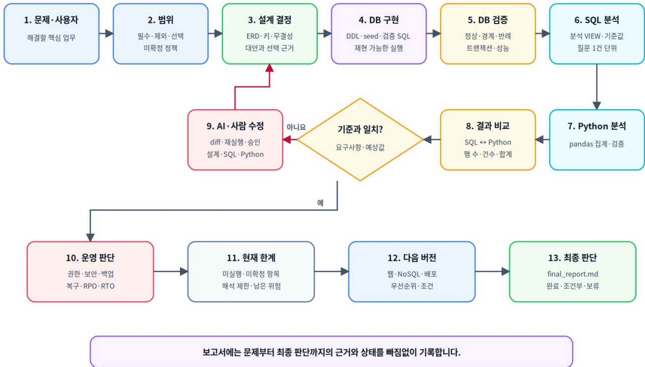
그림 15-7 설계 결정과 검증 근거를 설명하는 흐름
