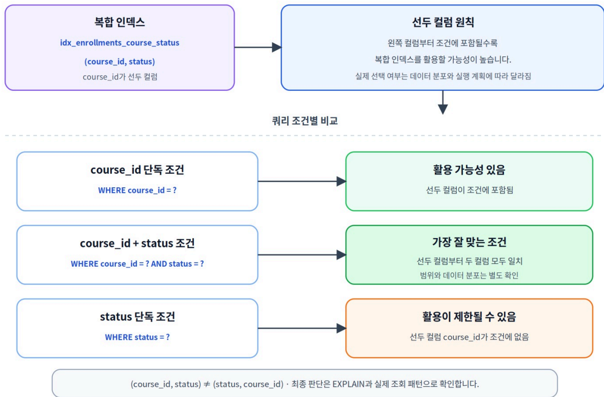
그림 10-5 복합 인덱스의 선두 컬럼과 쿼리 조건
