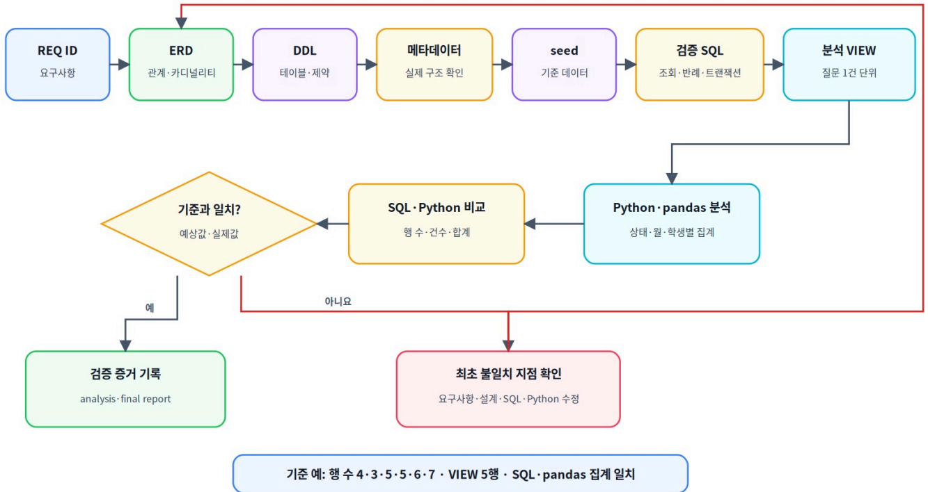
그림 15-4 요구사항부터 분석 결과까지 검증하기
