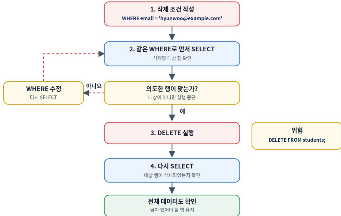
그림 4-7 안전한 DELETE 실행 절차
