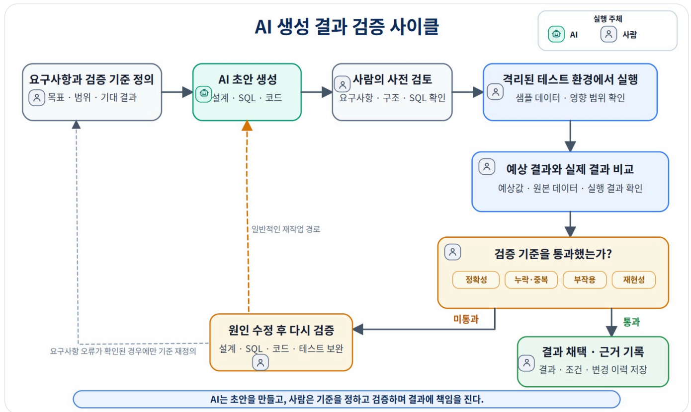
그림 1-2 AI 생성 결과 검증 사이클
