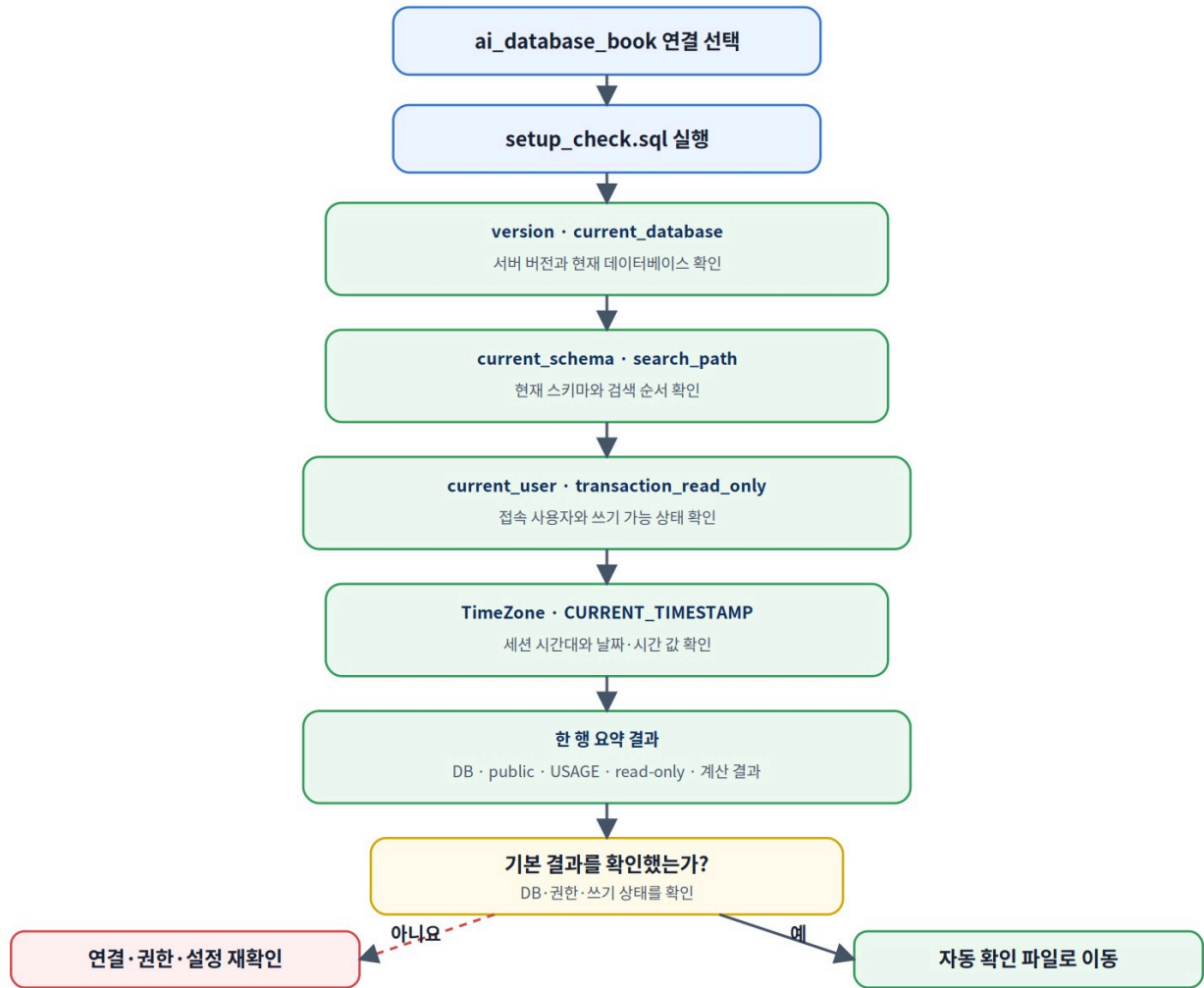
그림 3-4 SQL로 환경 정보 확인하기
