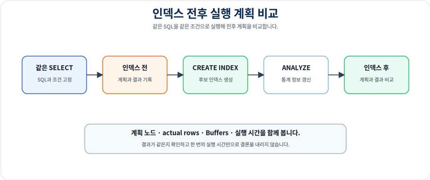
그림 10-7 인덱스 전후 실행 계획 비교
