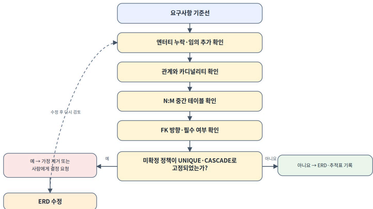
그림 13-4 요구사항을 기준으로 ERD 검토하기
