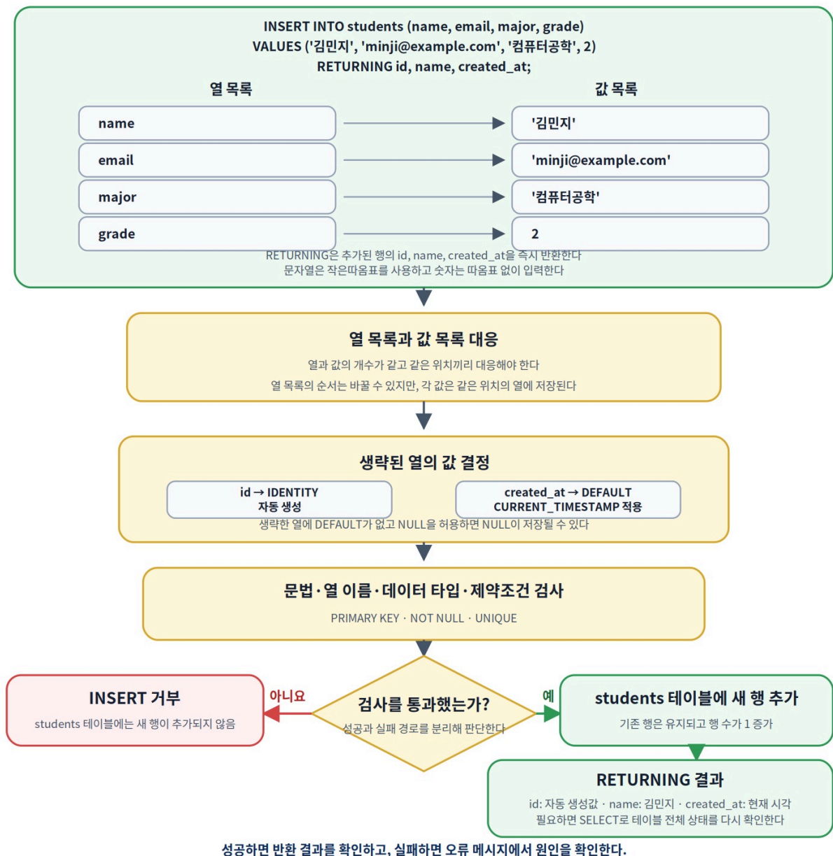
그림 4-2 INSERT로 새 행 추가하기
