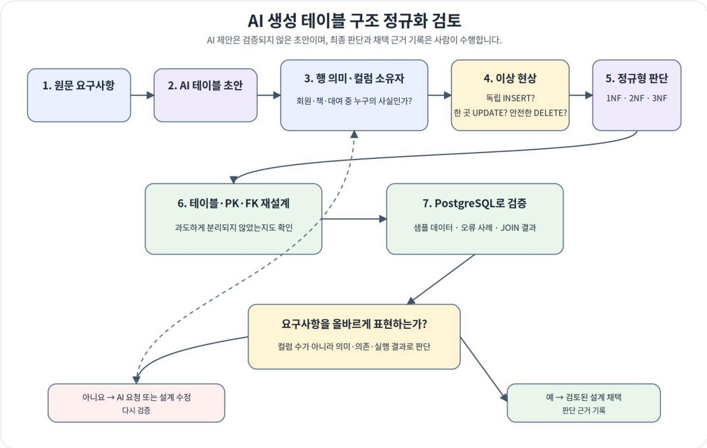
그림 6-8 AI 생성 구조와 무결성 검토 흐름
