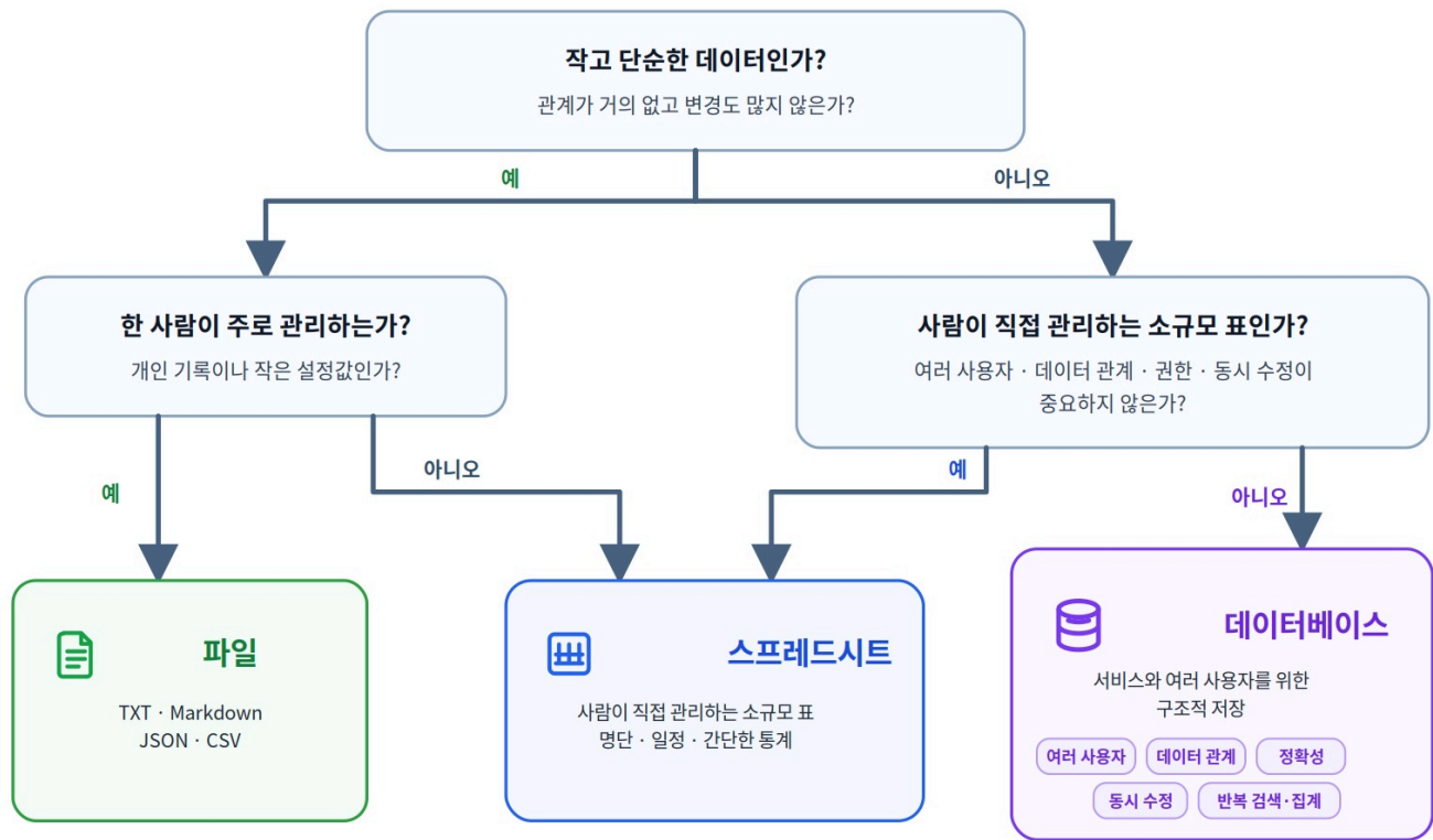
그림 1-1 데이터 특성에 따른 저장 방식 선택 흐름
