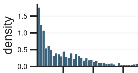
m3: Gauss+HRF
