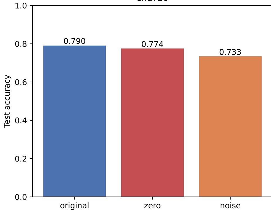
cifar10
