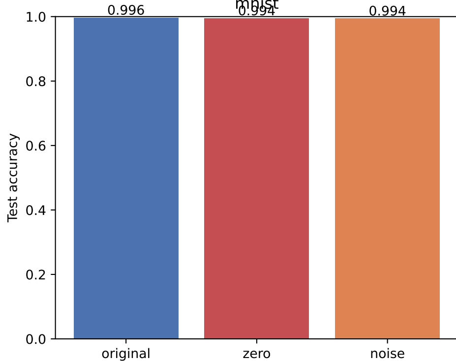
mnist
