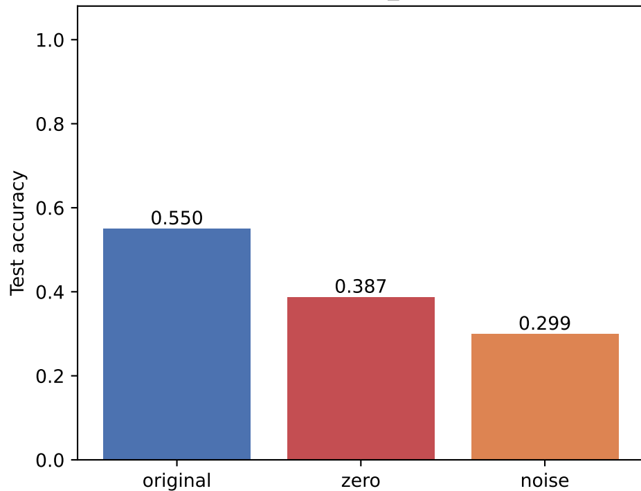
fer2013_hf
