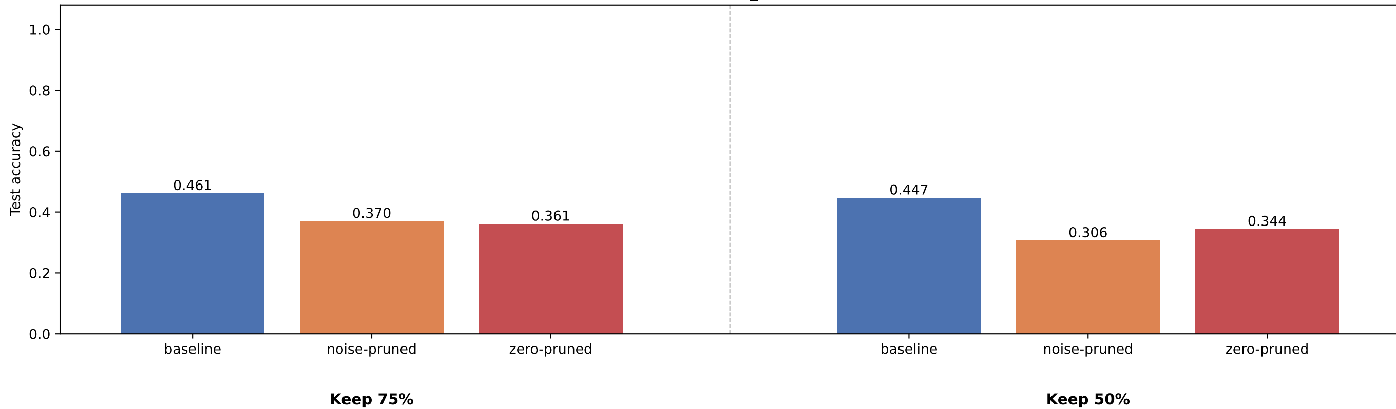
fer2013_hf
