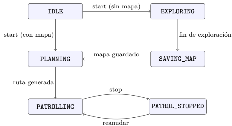
Figura 5.2: Transiciones de la máquina de estados del orquestador patrol_nav . El comando reinstall devuelve la FSM a IDLE desde cualquier estado. Fuente: elaboración propia.
