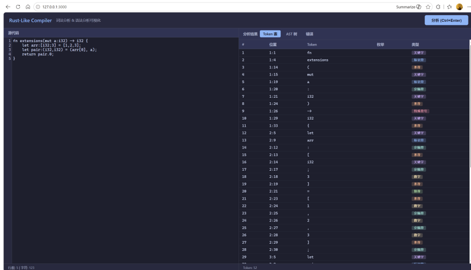
图 6: Web 页面中 token 展示设计
