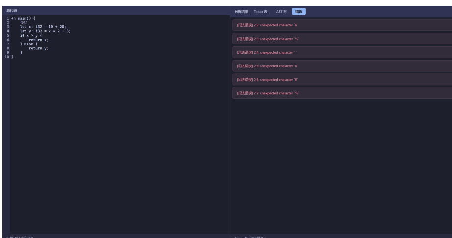
图 8: Web 页面中词法错误展示设计
