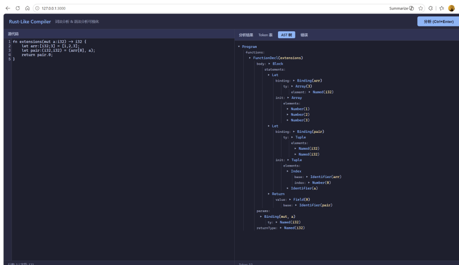
图 7: Web 页面中 AST 展示设计
