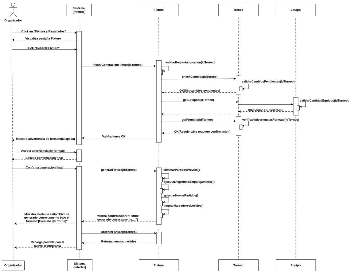
Figura 9. Diagrama de secuencia: Generar Fixture: Curso Normal
