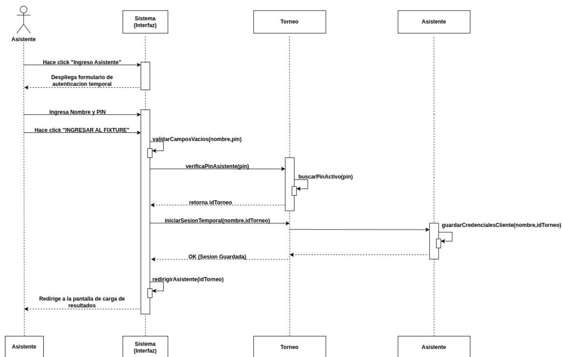
Figura 15. Diagrama de secuencia: Iniciar Sesión: Curso Normal
