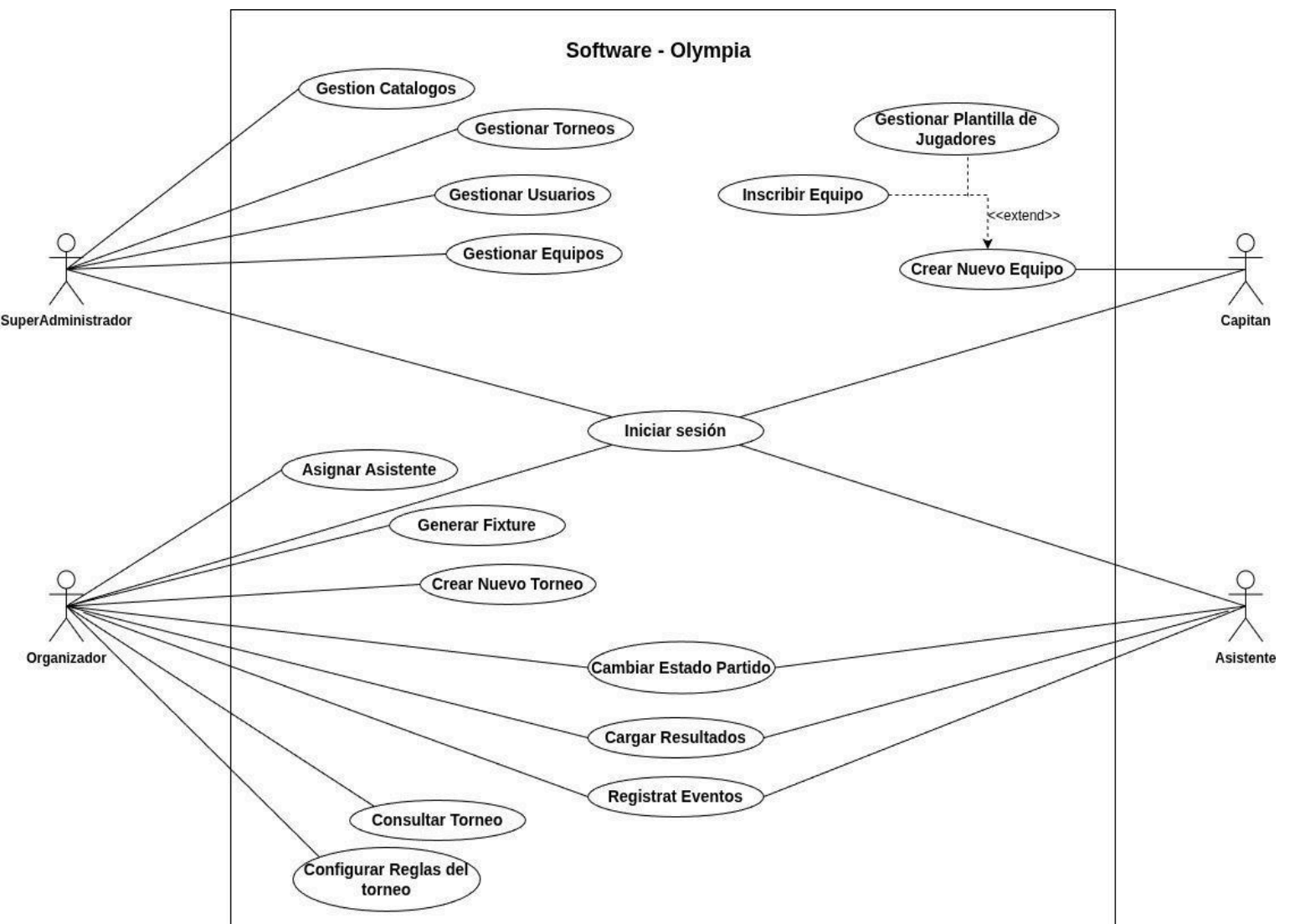
Figura 4. Caso de uso
