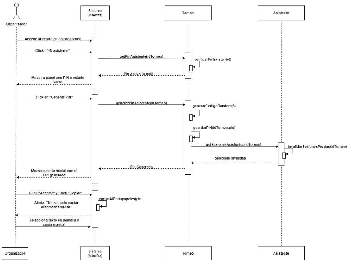
Figura 14. Diagrama de secuencia: Asignar Asistente: Curso Alternativo (Fallo de copia Automática)
