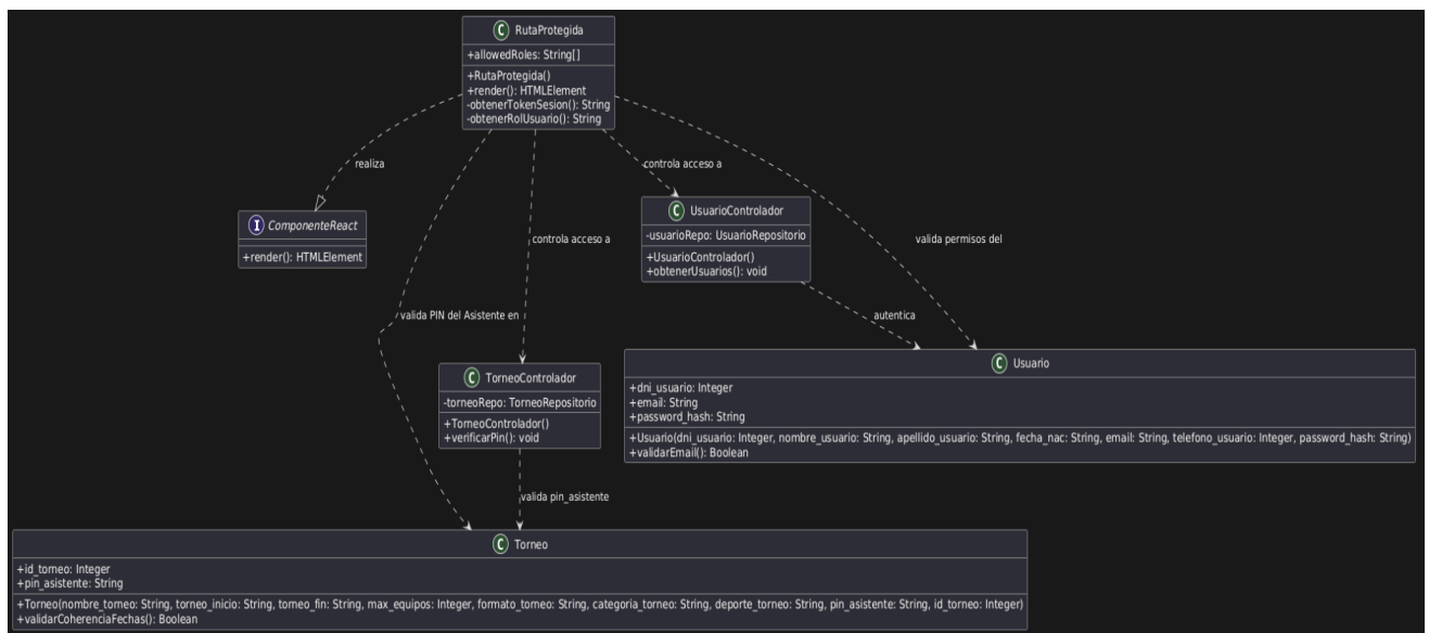
Figura 17. Patrón de implementación
