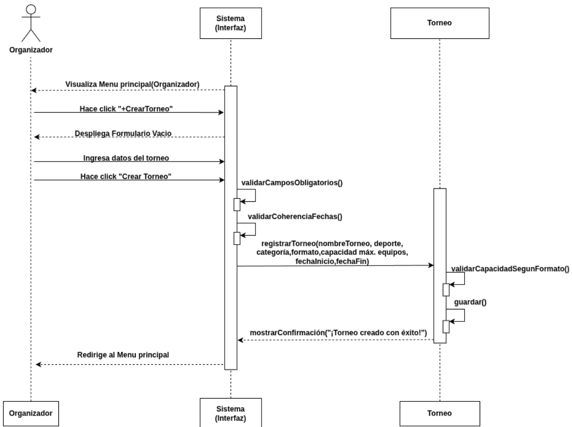
Figura 5. Diagrama de secuencia: Crear Nuevo Torneo: Curso Normal
