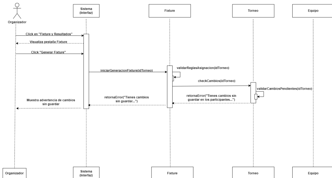
Figura 10. Diagrama de secuencia: Generar Fixture: Curso Alternativo (Cambios Pendientes)
