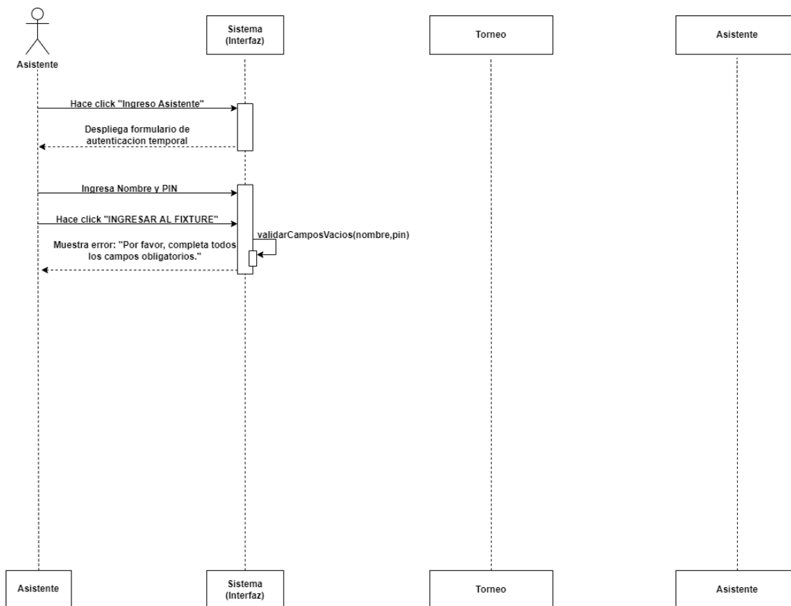
Figura 16. Diagrama de secuencia: Iniciar Sesión: Curso Alternativo (Campos Incompletos)
