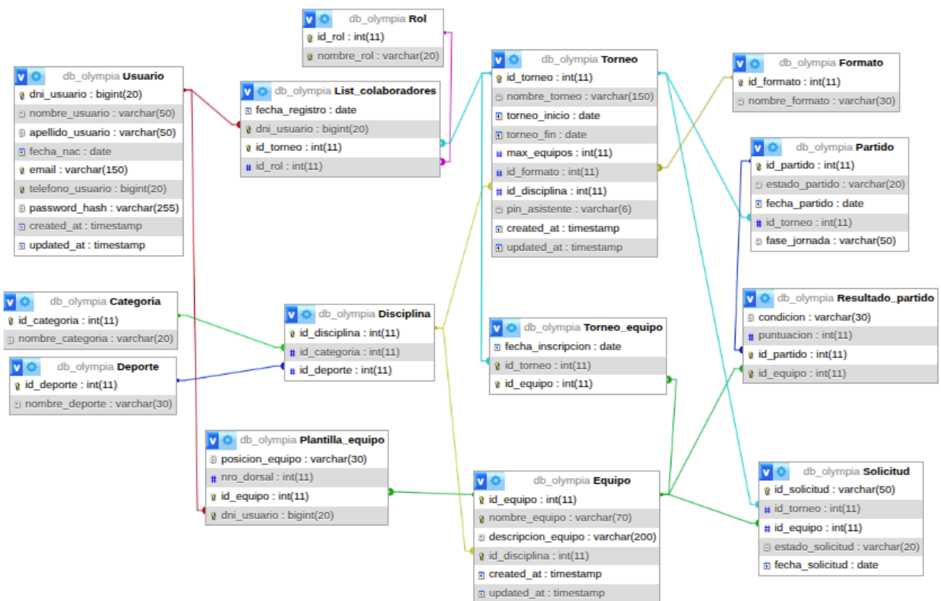
Figura 18. Diagrama Entidad Relación (DER)
