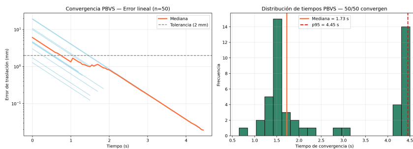
Figura 5. Convergencia del controlador PBVS sobre 50 poses reales de FoundationPose: curvas de error lineal (escala log) e histograma de tiempos de convergencia.
