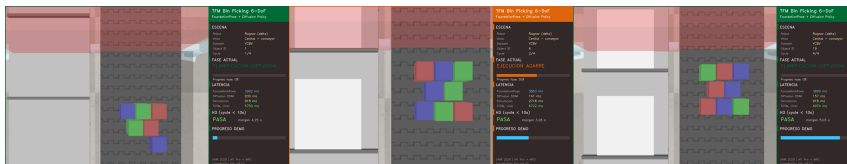
Figura 1. Tres frames del pipeline E2E ejecutado en CoppeliaSim Edu V4.10 (vista cenital del bin picking + panel de telemetría con latencias en tiempo real, fase actual y aceptación de H3). Cada columna corresponde a un ciclo distinto sobre objetos YCB-V ( obj_id =1, 6, 14).
