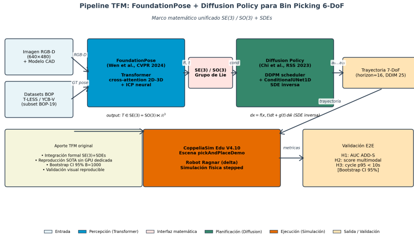
Figura 2. Diagrama de arquitectura del pipeline TFM con marco matemático unificado SE(3)/SO(3) + SDEs.
